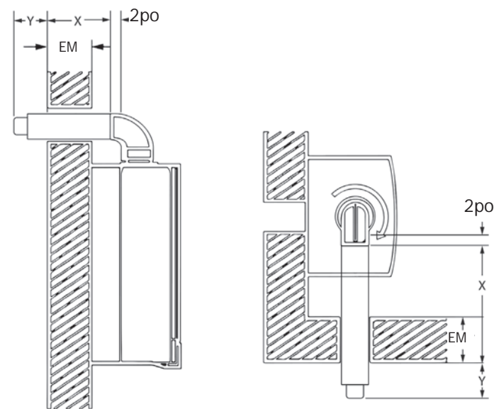
FIGURE 5-3– Événements coaxiaux horizontaux ou verticaux Peut Être Utilisé Sur Toutes les Grandeurs
