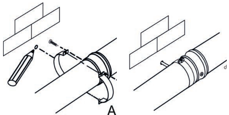
Figure 5-1 - Le fait de Décharger le Soutien
