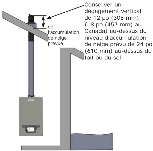
FIGURE 5-4 – Événement coaxial pour installation sur le toit Peut Être Utilisé Sur Toutes les Grandeurs
