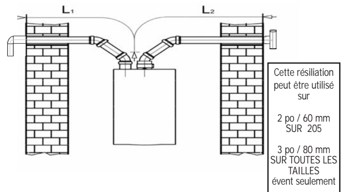
FIGURE 5-10 - 2po/ 60 mm* 3po/ 80 mm Twin Pipe Séparée Tuyau D’évacuation Horizontale Avec Té Sur Échappement - Peut Être Utilisé Sur Toutes les Grandeurs
