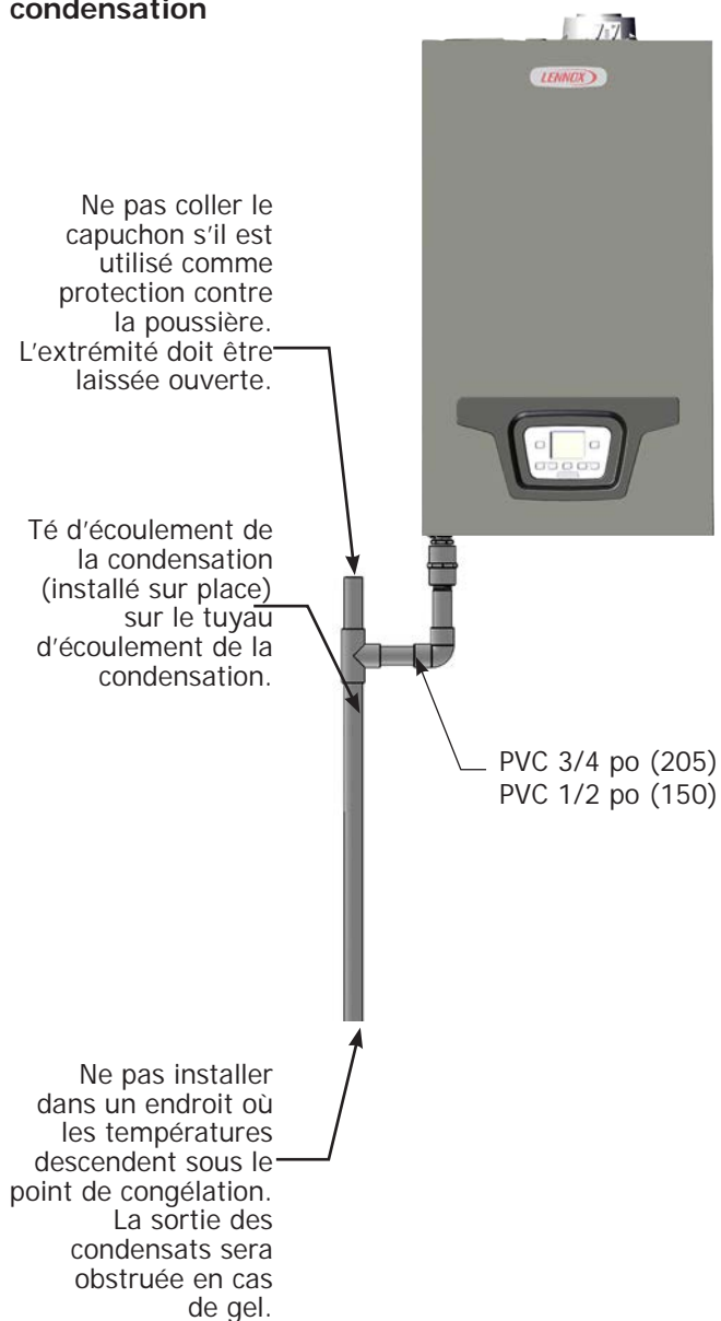
FIGURE 5-26 – Tuyau d'écoulement de la condensation
