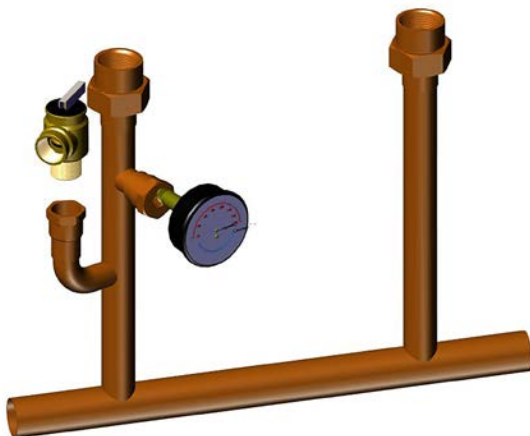
DISTRIBUTEUR GCWB95W-150/205
