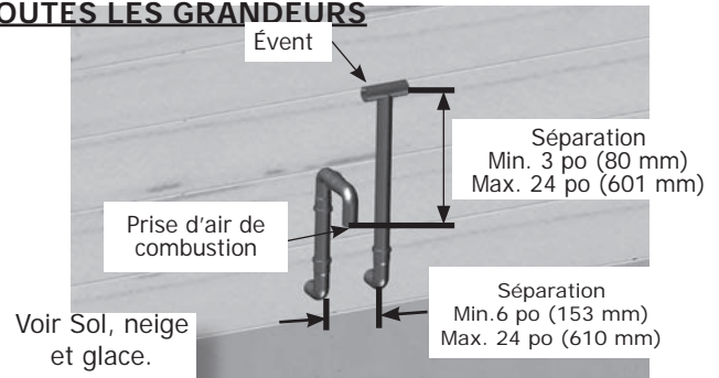
FIGURE 5-22 - (2po SEULEMENT) la Bouche de Côté de Pipe de Jumeau Muralet PEUT ÊTRE UTILISÉ SUR TOUTES LES GRANDEURS
