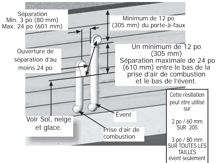
FIGURE 5-19 – (3 po/80 mm seulement) Évent latéral de tuyau double
