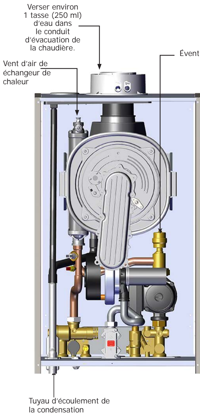
FIGURE 9-1 Module d'écoulement de la condensation Modèle 205 illustré (emplacement semblable pour toutes les dimensions)
