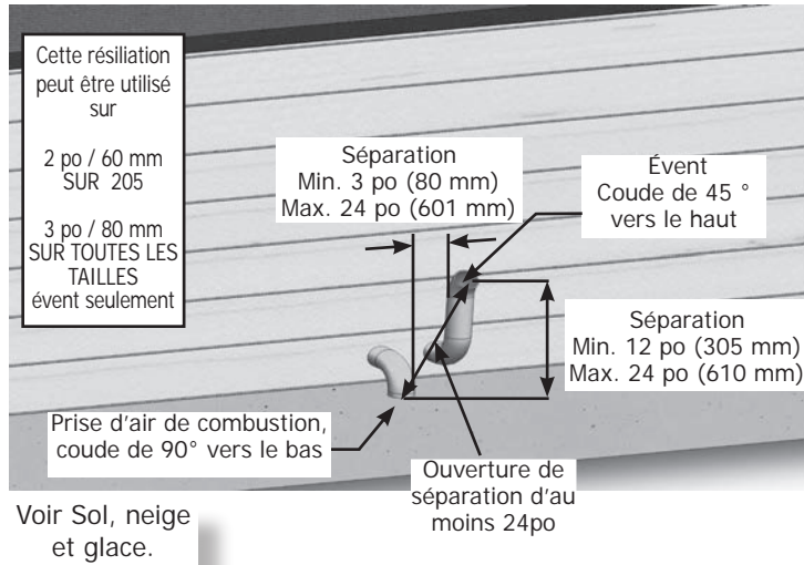
FIGURE 5-19 – (3 po/80 mm seulement) Évent latéral de tuyau double
