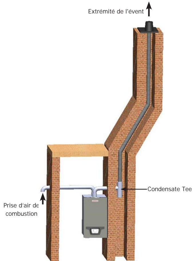
FIGURE 5-24 – (3po/ 80 mm seulement) Système d'évacuation flexible PEUT ÊTRE UTILISÉ SUR TOUTES LES GRANDEURS
