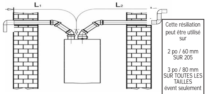
FIGURE 5-10 - 2po/ 60 mm* 3po/ 80 mm Twin Pipe Séparée Tuyau D’évacuation Horizontale Avec Té Sur Échappement - Peut Être Utilisé Sur Toutes les Grandeurs
