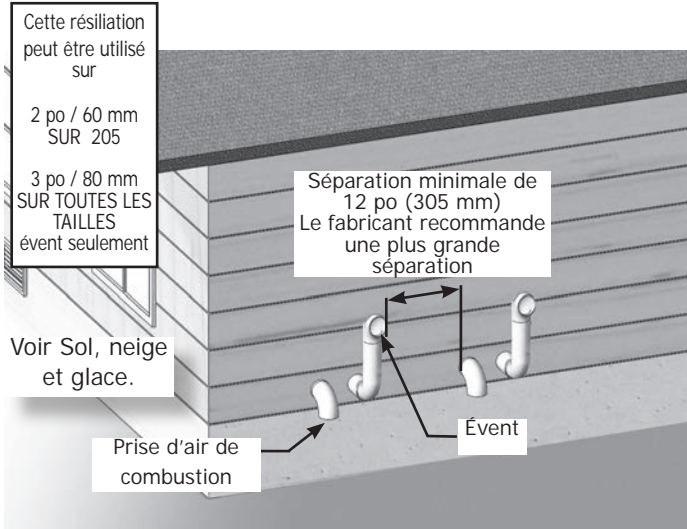
FIGURE 5-18 – (3 po/80 mm seulement) Évent latéral de tuyau double avec angle de 45°
