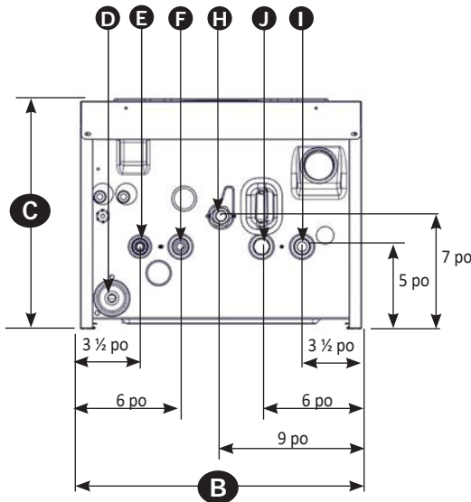
150 COMBI Vue de dessous Dimensions
