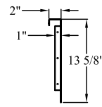
VERTI. SCOOP PIECE (x1)
