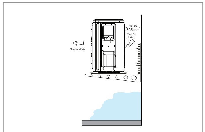
Figure 16. Unité extérieure sur supports au-dessus du niveau de la neige
