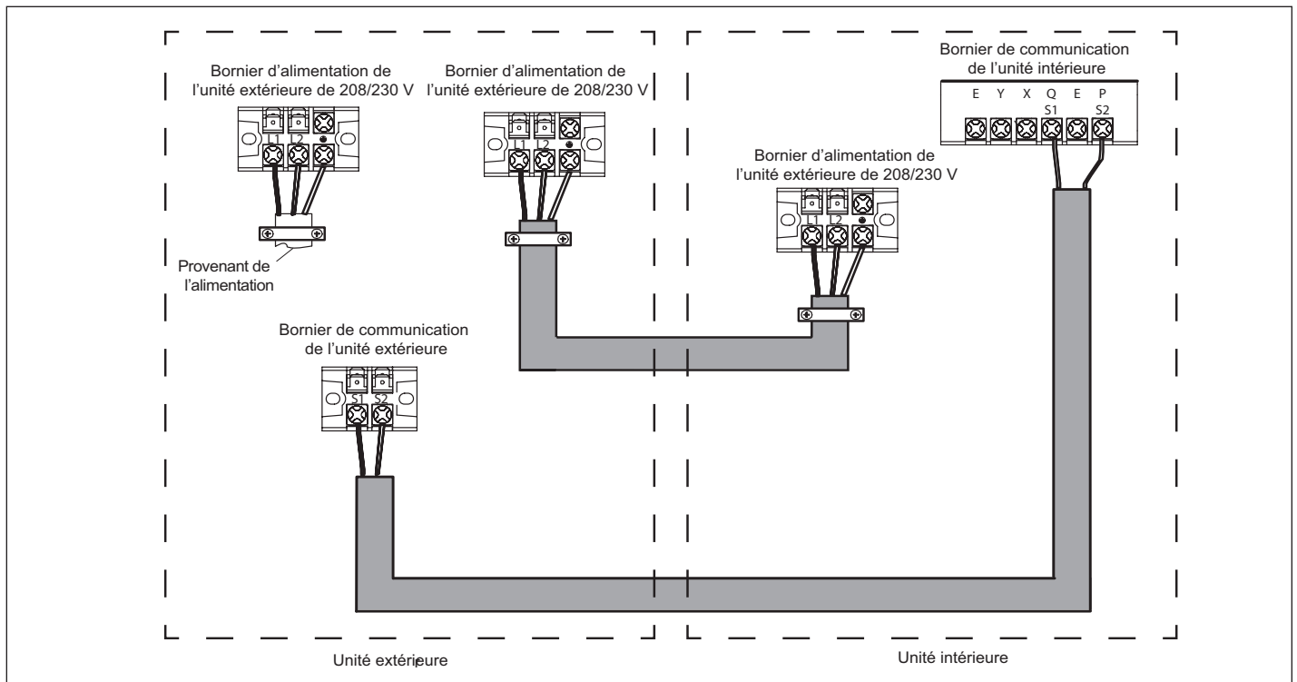
Figure 30. Câblage simple zone 36K et plus
