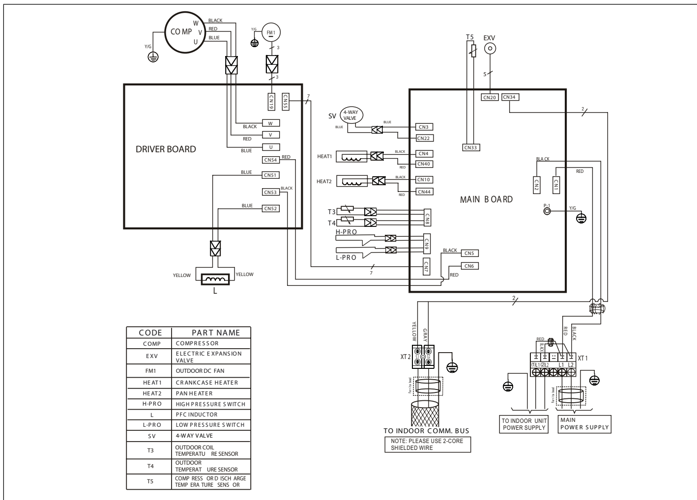
Figure 36. Schéma de câblage de l'unité extérieure 208/230V MPB036S4S-*P
