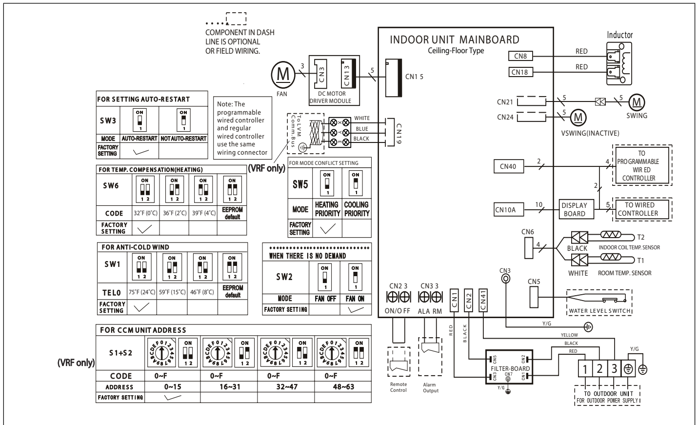
Figure 31. Schéma de câble de l'unité MCFB018S4*P
