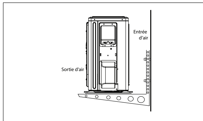
Figure 25. Fixation de l'unité extérieure sur des équerres
