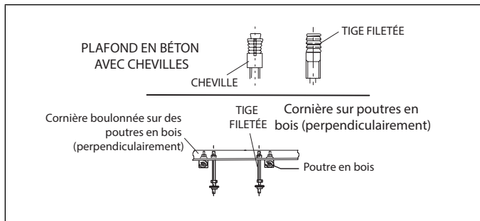
Figure 11. Emplacement des tiges filetées
