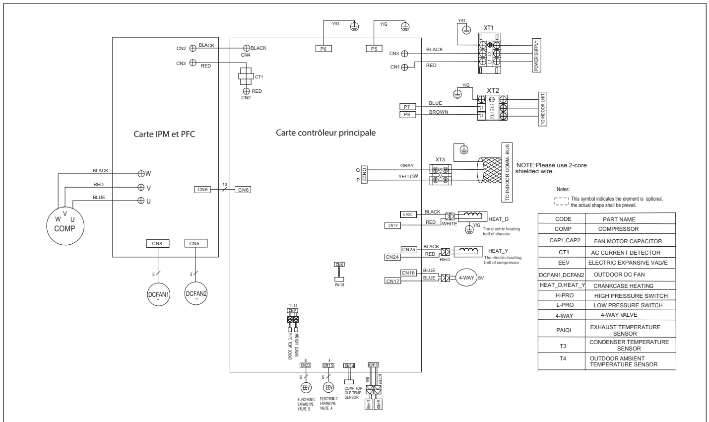
Figure 39. Schéma de câblage de l'unité extérieure 208 / 230V MLB036S4S- * P et MLB048S4S- * P
