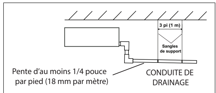
Figure 13. Unité intérieure suspendue au plafond utilisant un drain par gravité de pente correcte
