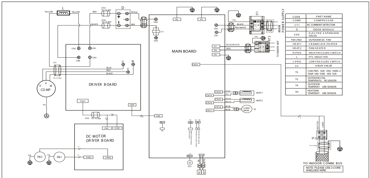
Figure 37. Schéma de câblage de l'unité extérieure 208/230V MPB048S4S-*P
