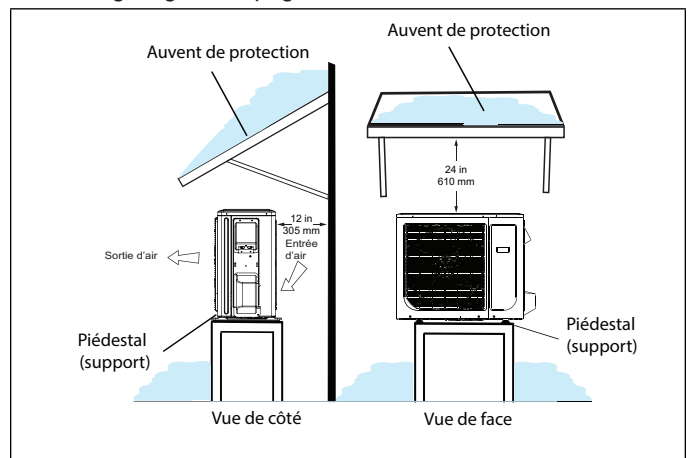
Figure 15. Unité extérieure sur piédestal et sous auvent de protection
