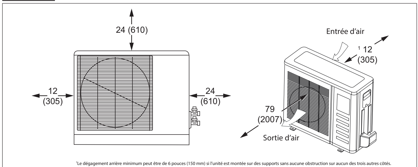
Figure 5. Dégagements de l'unité extérieure - pouces (mm)
