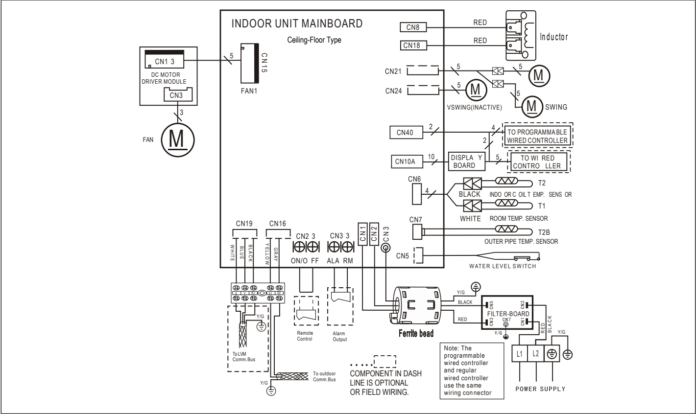
Figure 34. Schéma de câblage de l'unité MCFA048S4-*P
