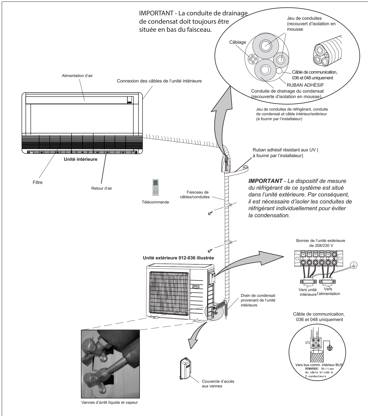
Figure 1. Système typique illustré
