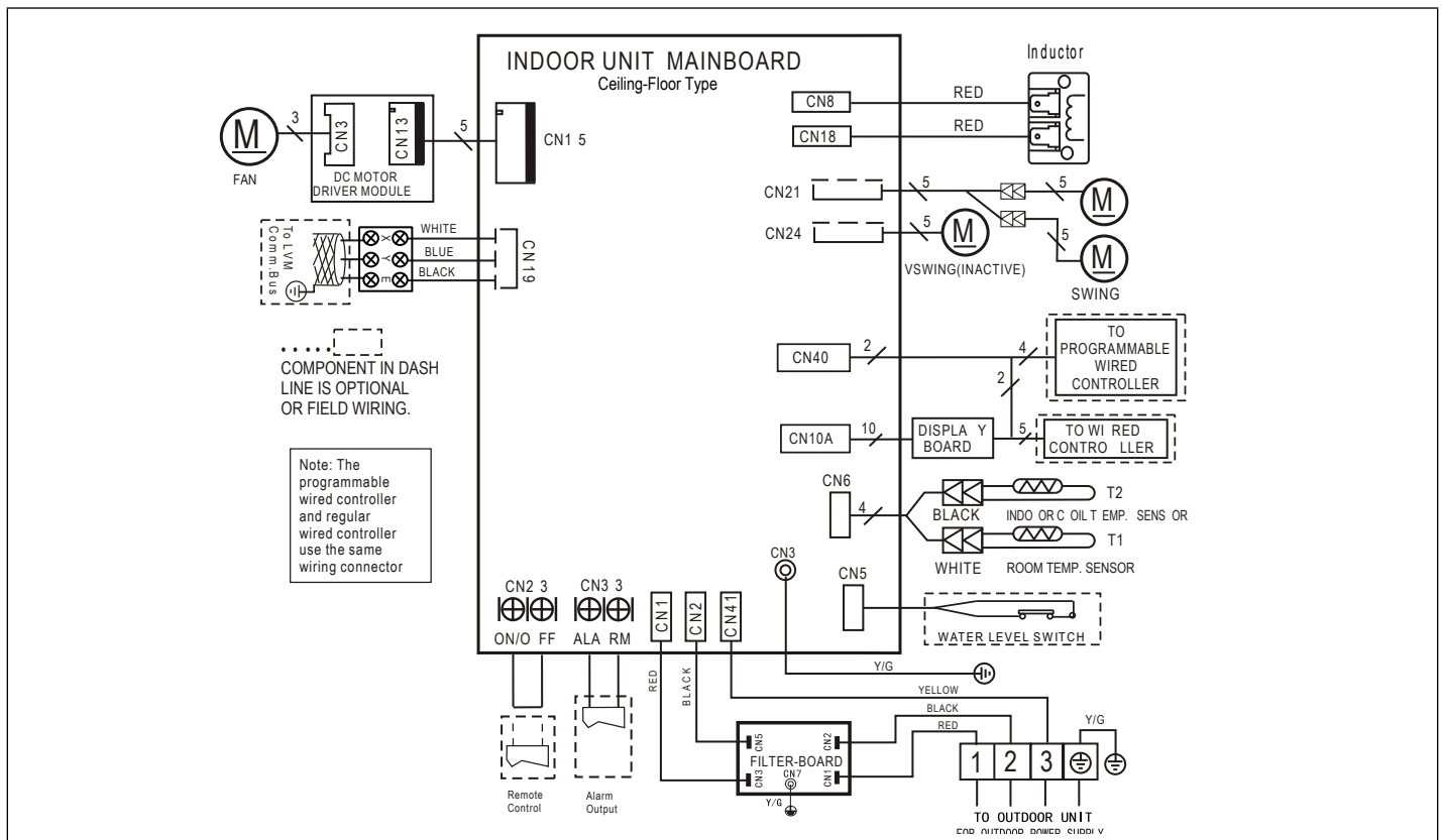
Figure 32. Schéma de câblage de l'unité MCFA024S4*P
