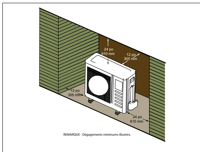
Figure 21. Unité installée dans une alcôve
