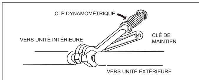
Figure 28. Serrer l'écrou évasé
