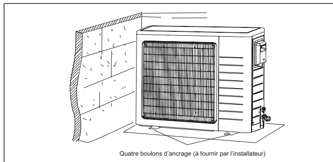
Figure 23. Fixation de l'unité extérieure sur une dalle
