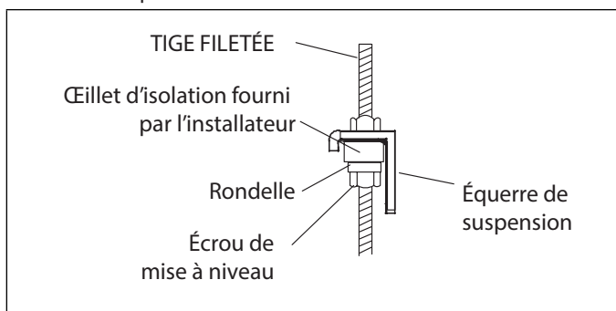
Figure 12. Emplacement du support sur la tige filetée
