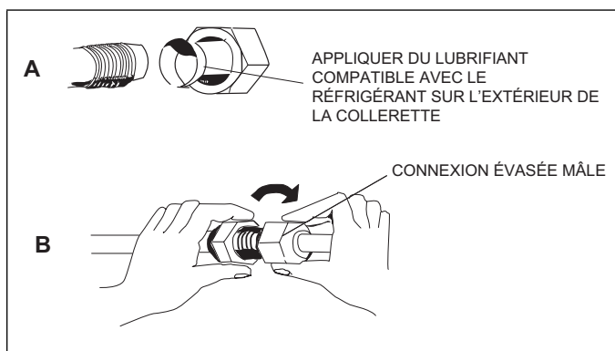
Figure 27. Réalisation des connexions mâles-femelles
