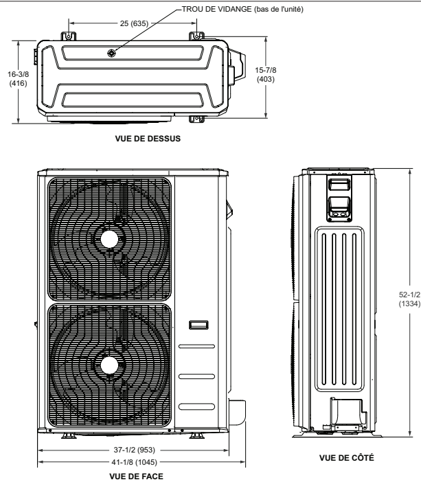
Figure 3. Dimensions de l'unité extérieure (MLB036S4S-* P, MLB048S4S-* P et MPB048S4S-* P - pouces (mm))
