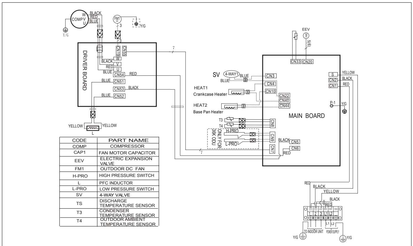
Figure 38. Schéma de câblage de l'unité extérieure 208/230V MLA024S4S-*P
