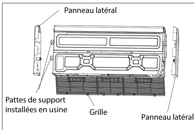
Figure 8. Retrait du panneau latéral et de la grille
