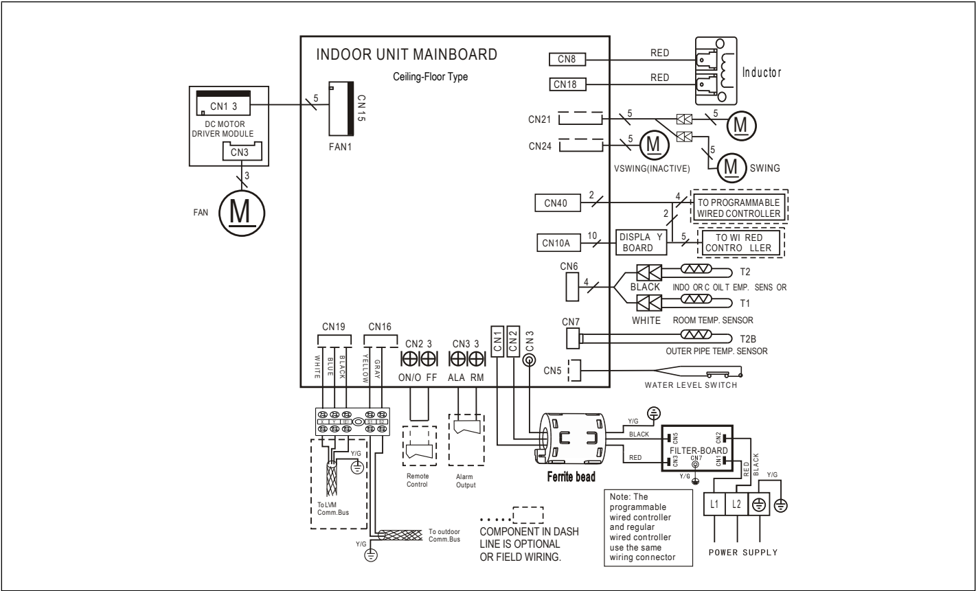
Figure 33. Schéma de câblage de l'unité MCFA036S4-*P
