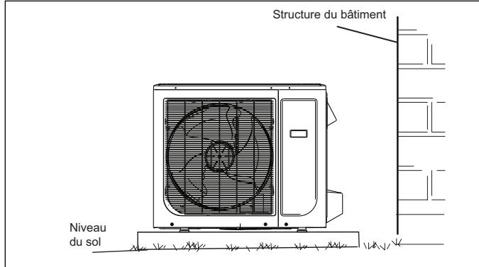
Figure 14. Installer l'unité de niveau (horizontale)
