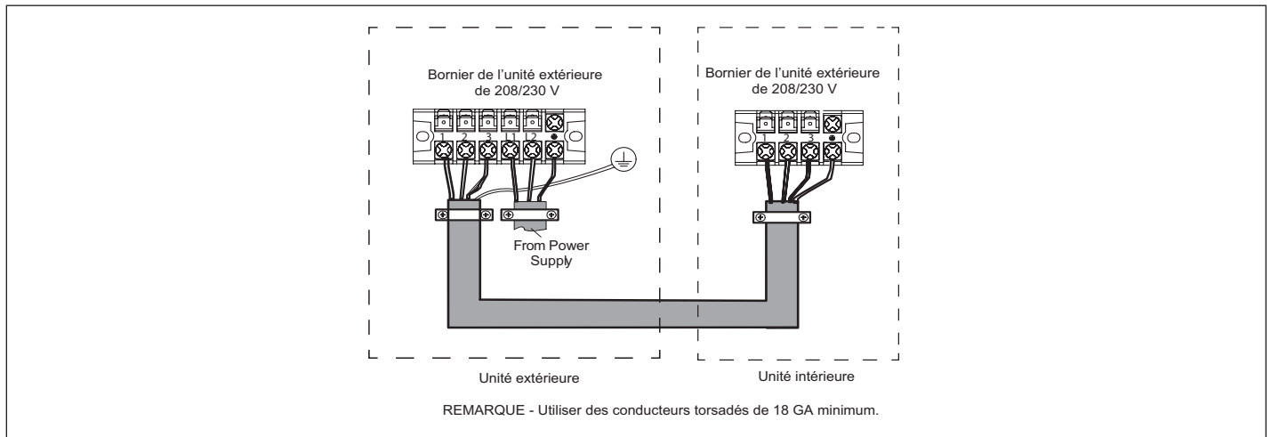
Figure 29. Câblage simple zone 30K et moins
