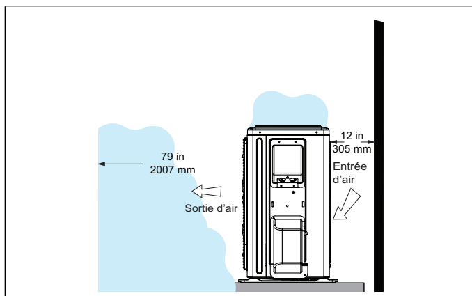
Figure 17. Débit d'air d'une unité extérieure obstrué par de la neige
