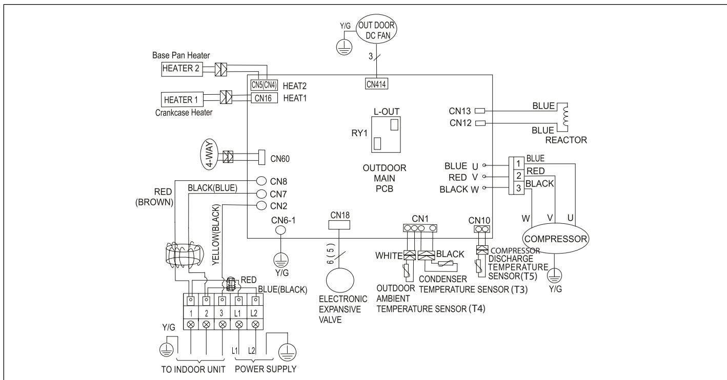
Figure 35. Schéma de câblage des unités extérieures 208/230V MPB018S4S-*P et MPB024S4S-*P
