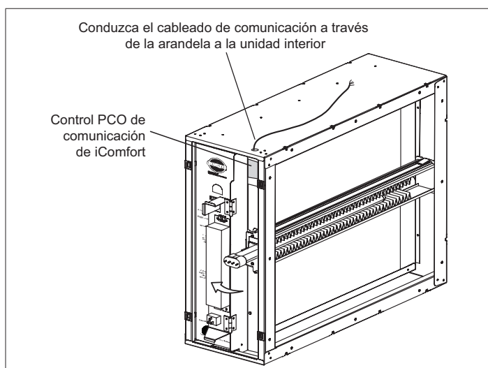
Figura 11. Ruta del cableado de comunicación
