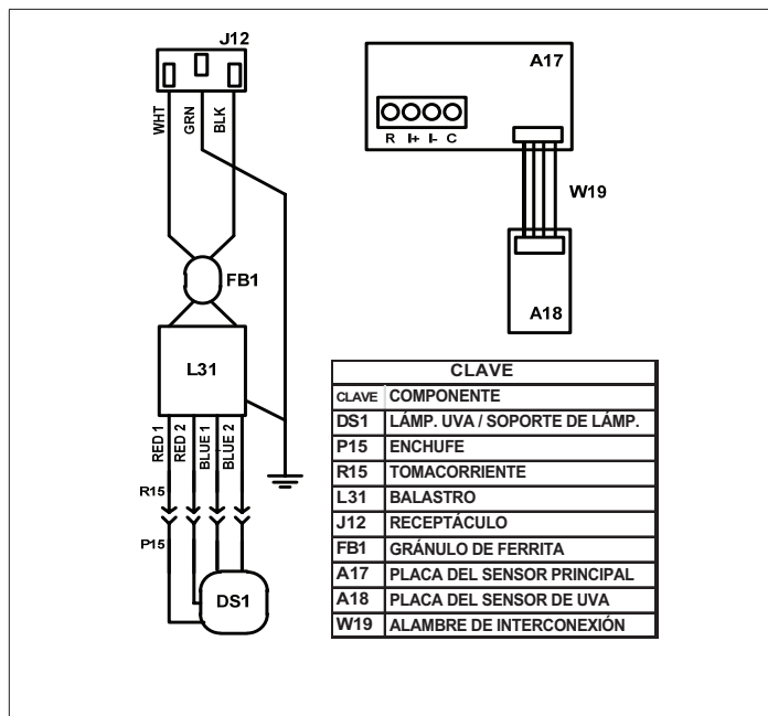
Figura 12. Diagrama esquemático de cableado del PCO
