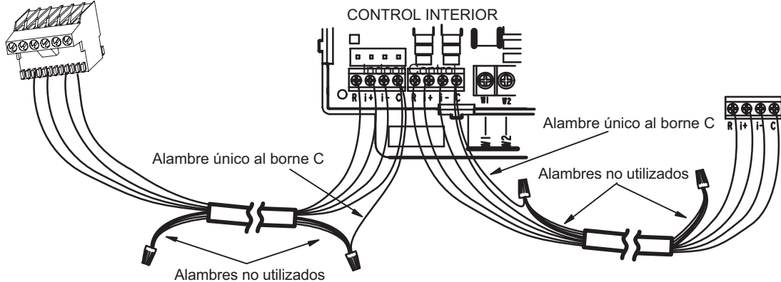
FIGURA 13. EL18XCV con termostato iComfort S30 con comunicación – Diagrama de cableado en el sitio
