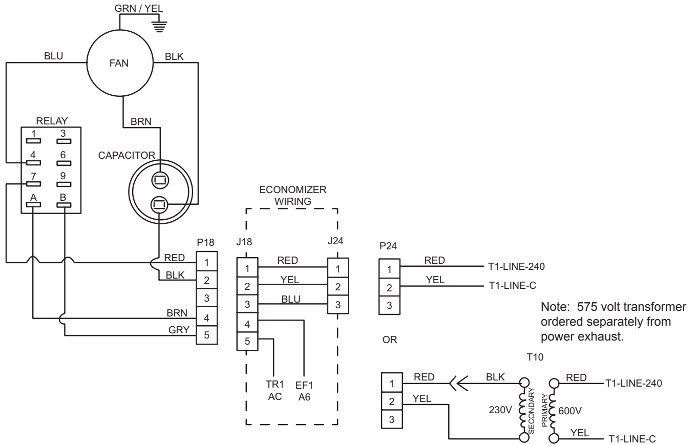
Figure 8 - Wiring Diagram for 230 volt and 575 volt
