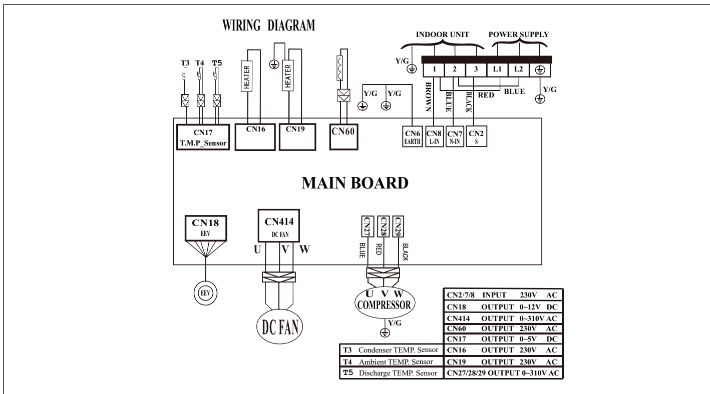
Figure 45. Schéma de câblage de l'unité extérieure 208/230V MPC024S4S-*P
