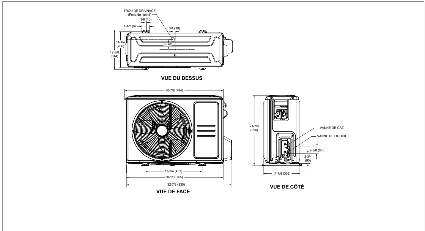
Figure 2. MPC009S4S-*P et MPC012S4S-*P - Dimensions de l'unité - pouces (mm)
