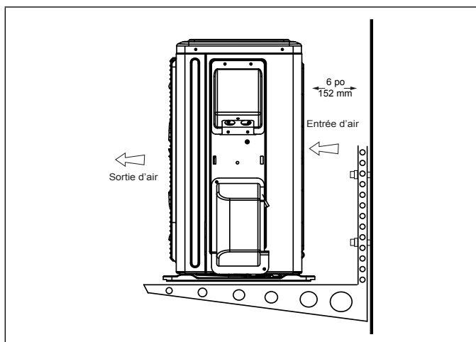
Figure 34. Fixation de l'unité extérieure sur des équerres
