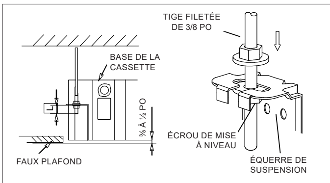
Figure 15. Matériel de suspension
