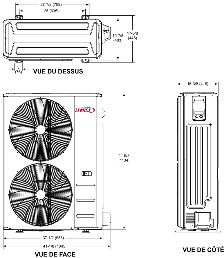
Figure 9. MLB036S4S-*P et MLB048S4S-*P - Dimensions de l'unité - pouces (mm)
