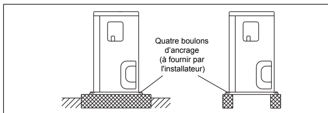
Figure 33. Fixation de l'unité extérieure sur des rails
