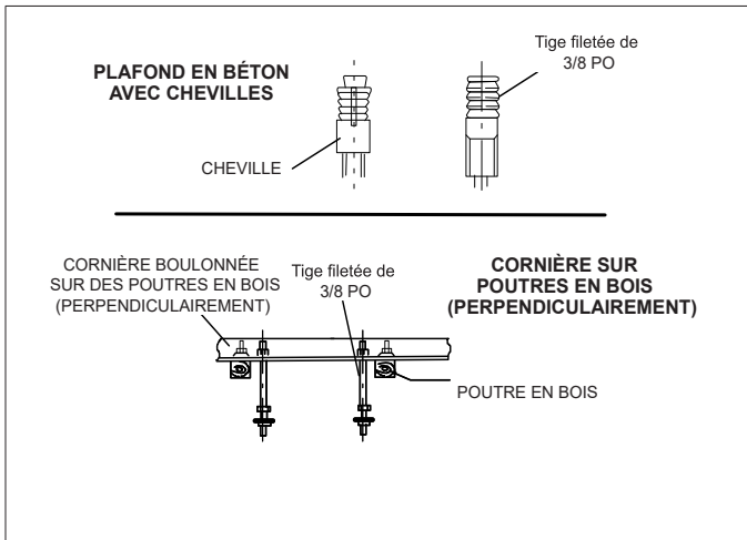
Figure 14. Méthodes de suspension
