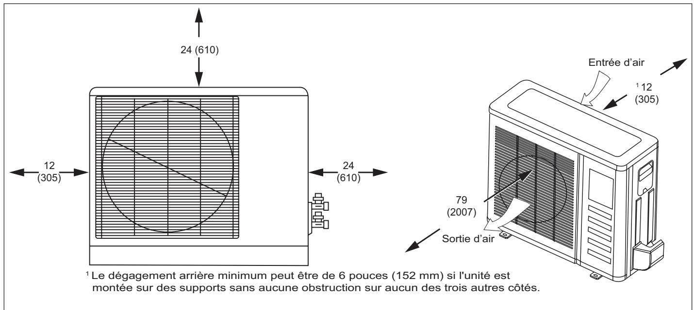
Figure 12. Dégagements de l'unité extérieure - pouces (mm)
