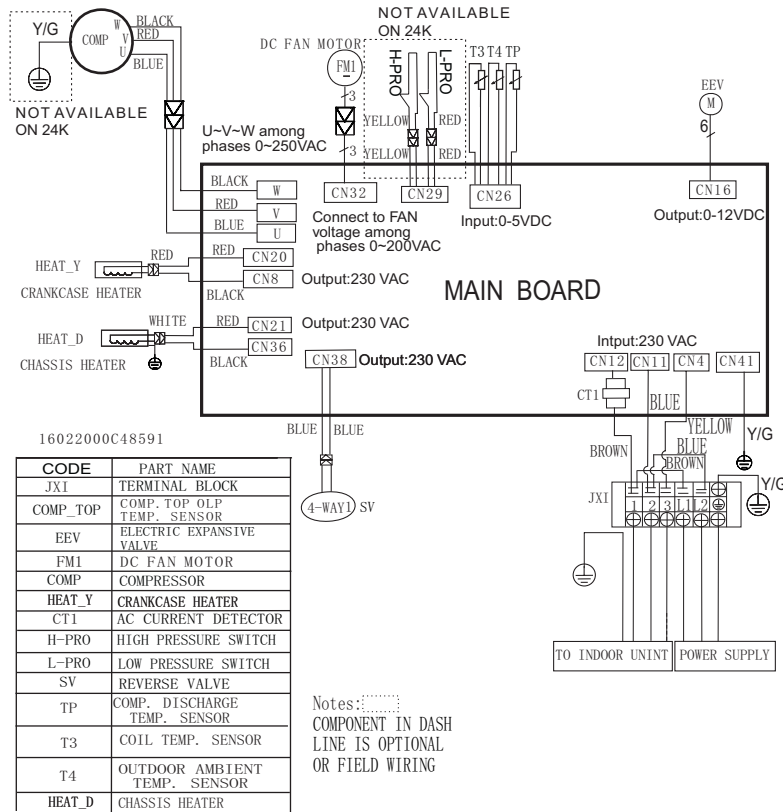
Figure 50. Schéma de câblage de l'unité extérieure 208/230V MLB024S4S-*P
