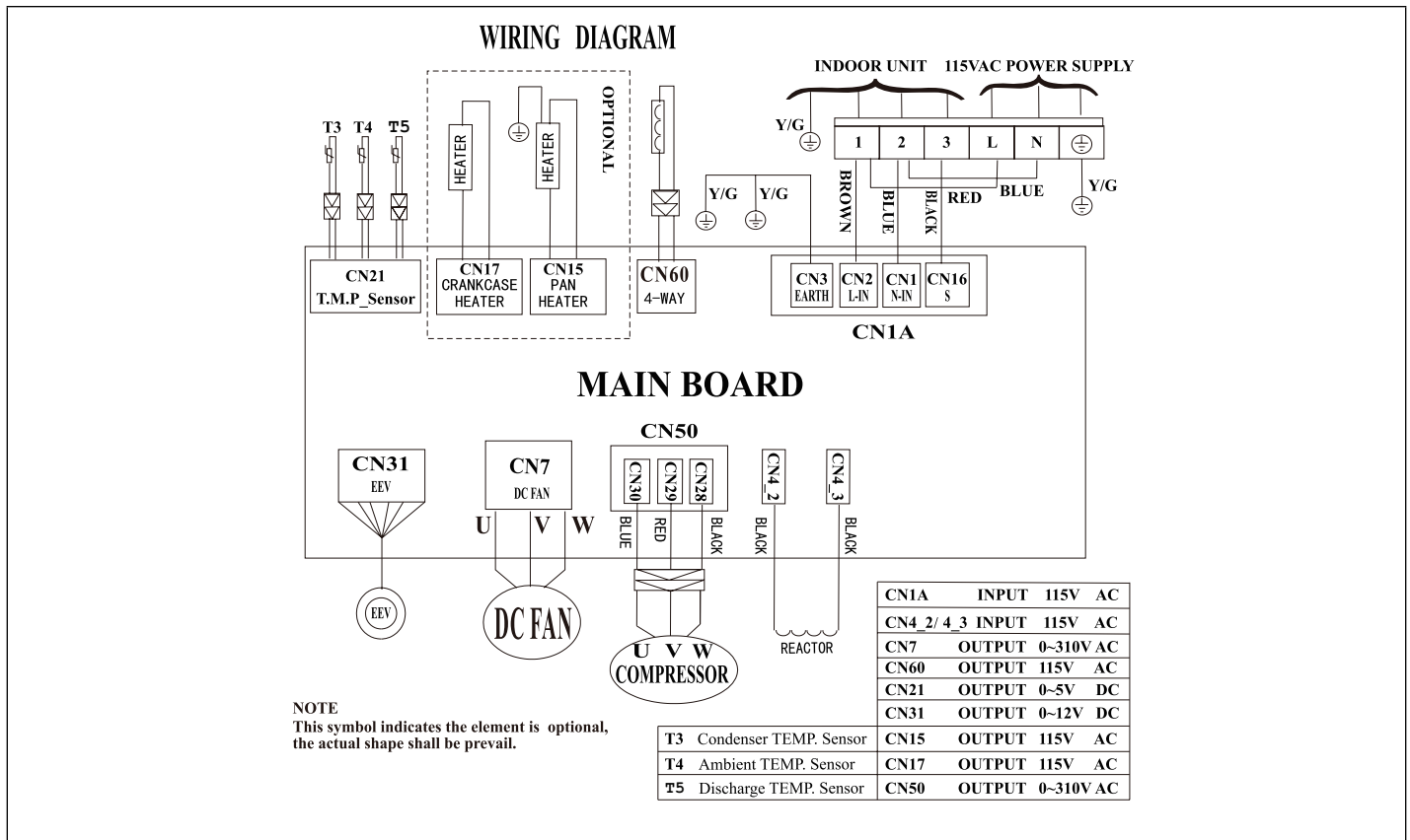
Figure 43. Schéma de câblage de l'unité extérieure 208/230V MPC012S4S-*P
