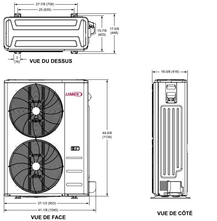
Figure 5. MPC048S4S-*P - Dimensions de l'unité - pouces (mm)
