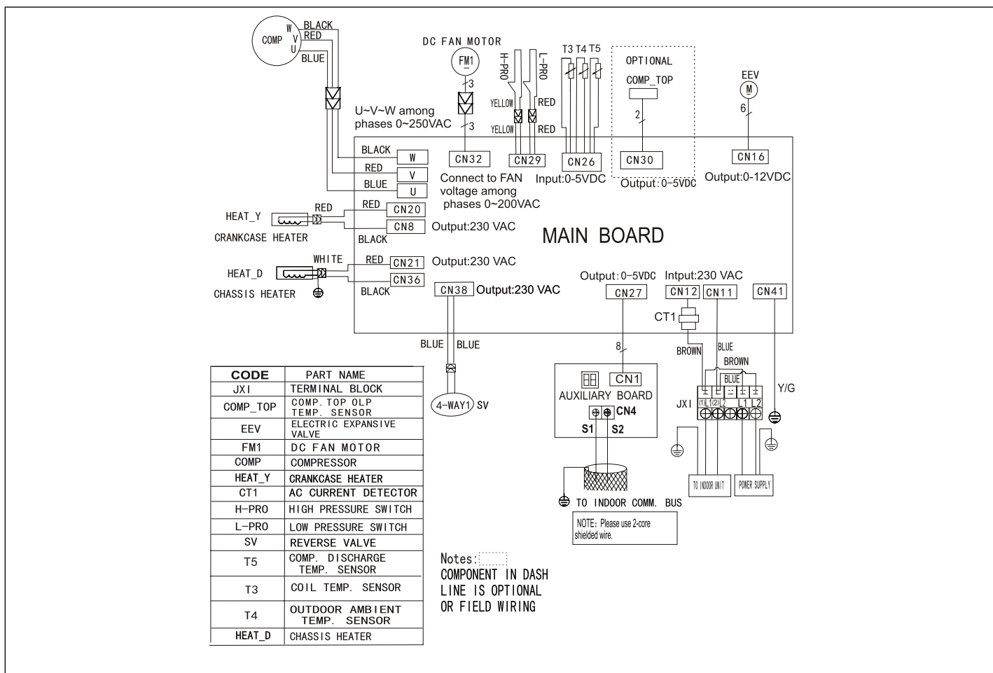
Figure 46. Schéma de câblage de l'unité extérieure 208/230V MPC036S4S-*P
