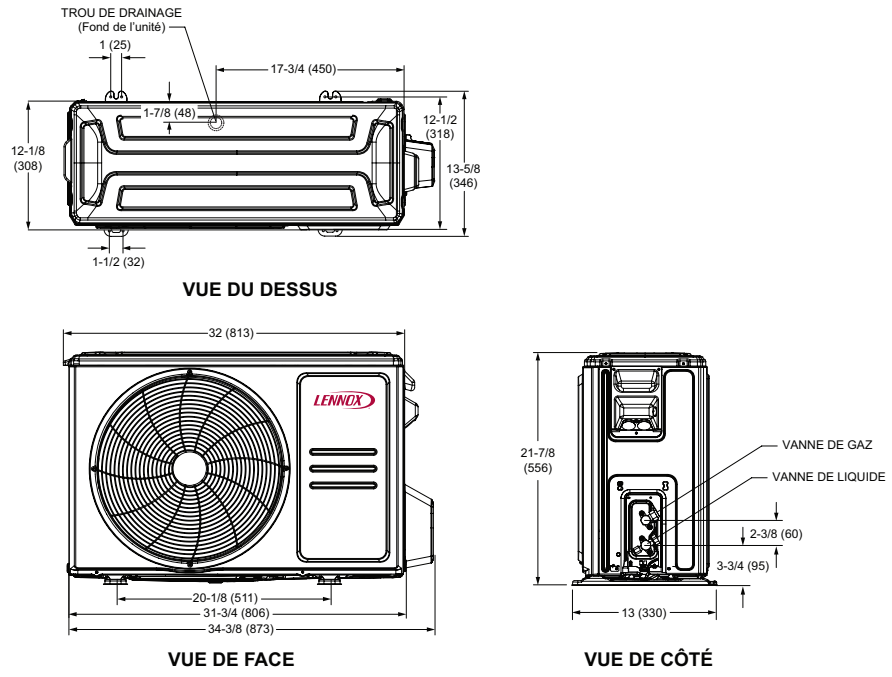
Figure 6. MLB009S4S-*P et MLB012S4S-*P - Dimensions de l'unité - pouces (mm)
