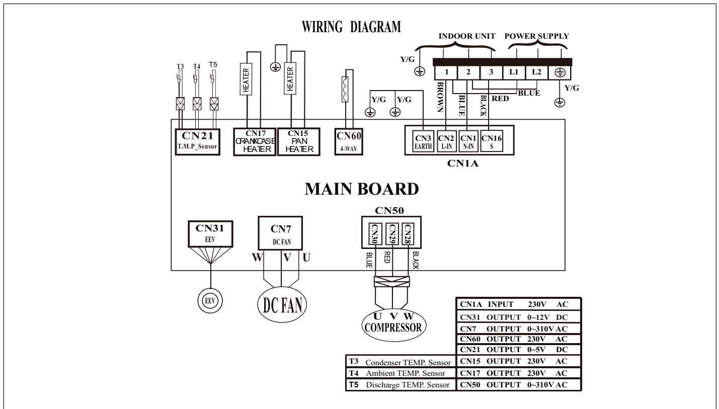
Figure 48. Schéma de câblage des unités extérieures 208/230V MLB009 et MLB0012S4S-*P
