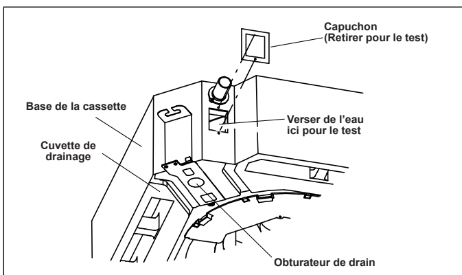
Figure 21. Test du drain de condensat
