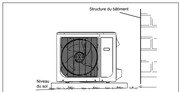
Figure 23. Installer l'unité de niveau (horizontale)
