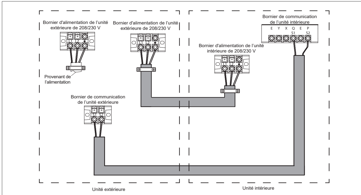
Figure 39. Câble simple zone 36K et 48K seulement
