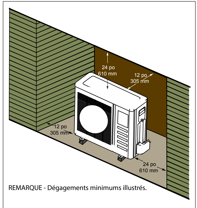
Figure 30. Unité installée dans une alcôve
