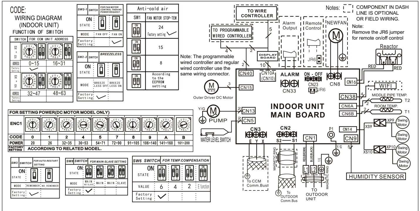
Figure 41. Schéma de câblage de l'unité M33C (toutes les puissances)
