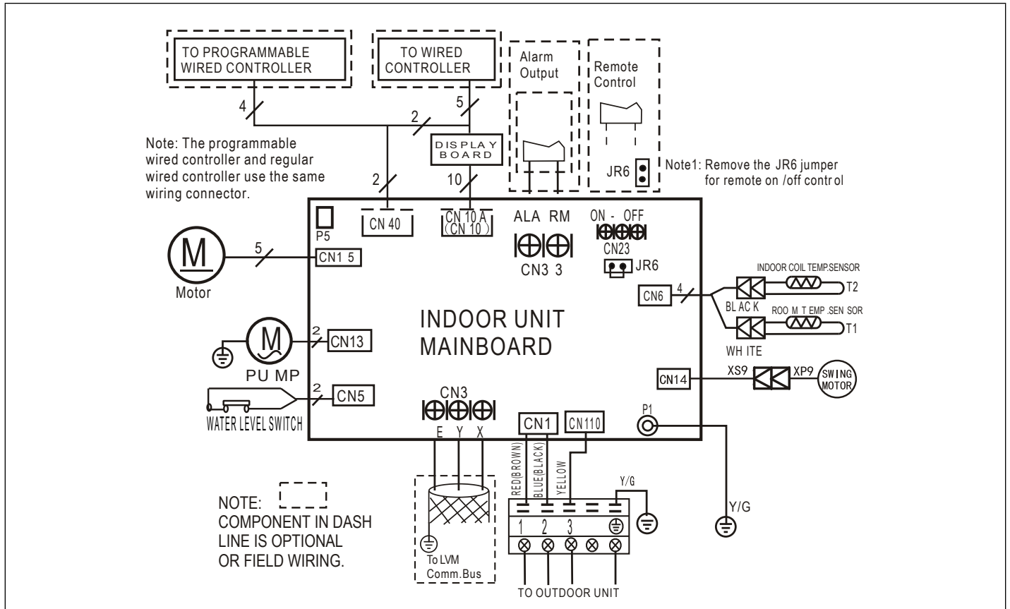
Figure 40. M22A018S4 Schéma de câblage des unités M22A009S4-*P, M22A012S4-*P et M22A018S4-*P
