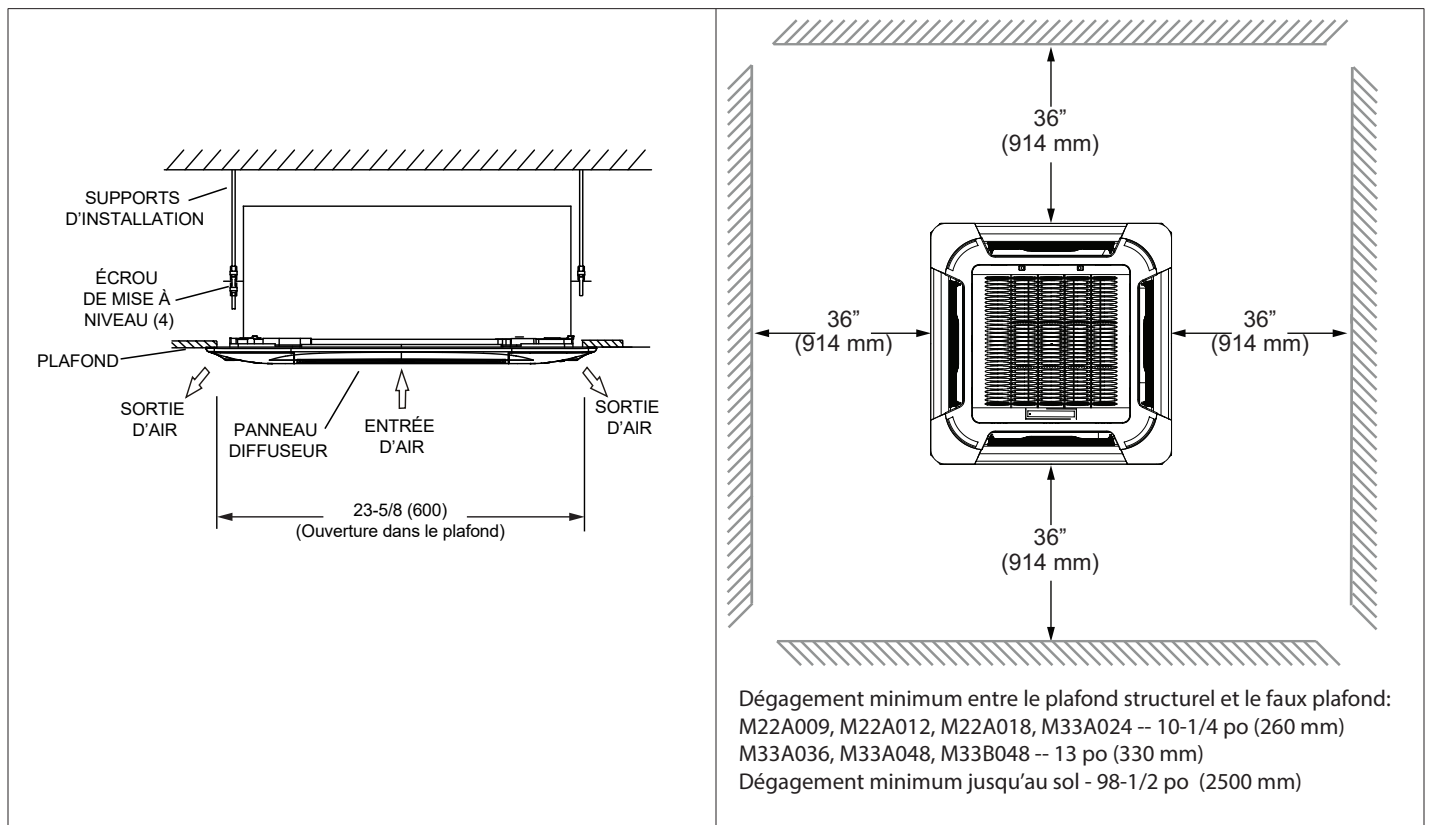
Figure 13. Dégagements pour l'unité intérieure - M22A et M33C - pouces (mm)
