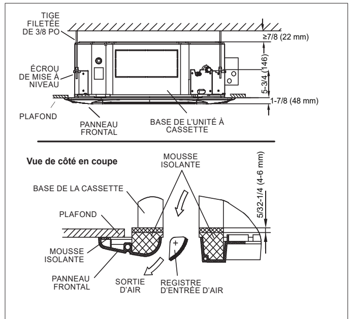
Figure 19. Panneau frontal en place
