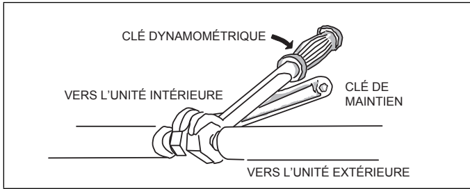
Figure 37. Serrer l'écrou évasé
