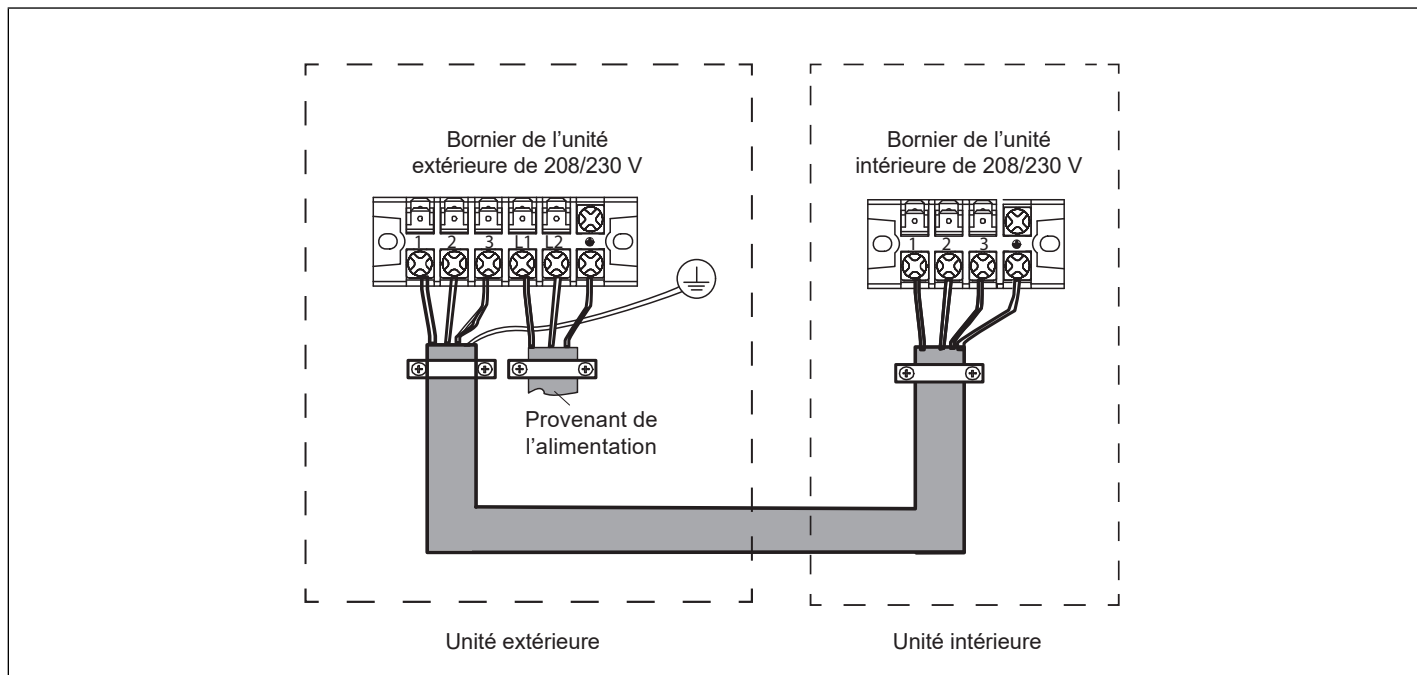
Figure 38. Câblage simple zone (09K à 24K)
