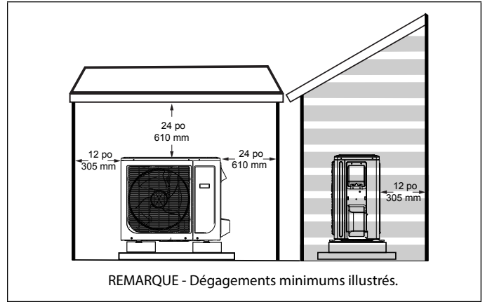
Figure 29. Abri de style niche à chien
