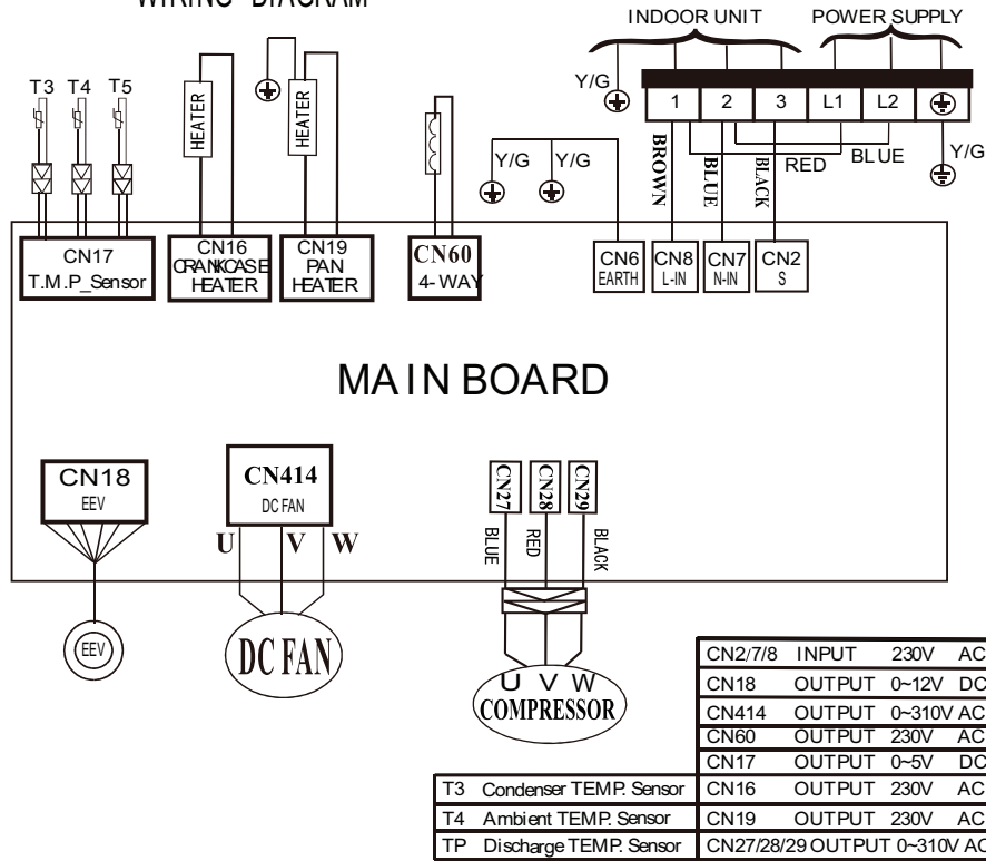
Figure 49. Schéma de câblage de l'unité extérieure 208/230V MLB0018S4S-*P
