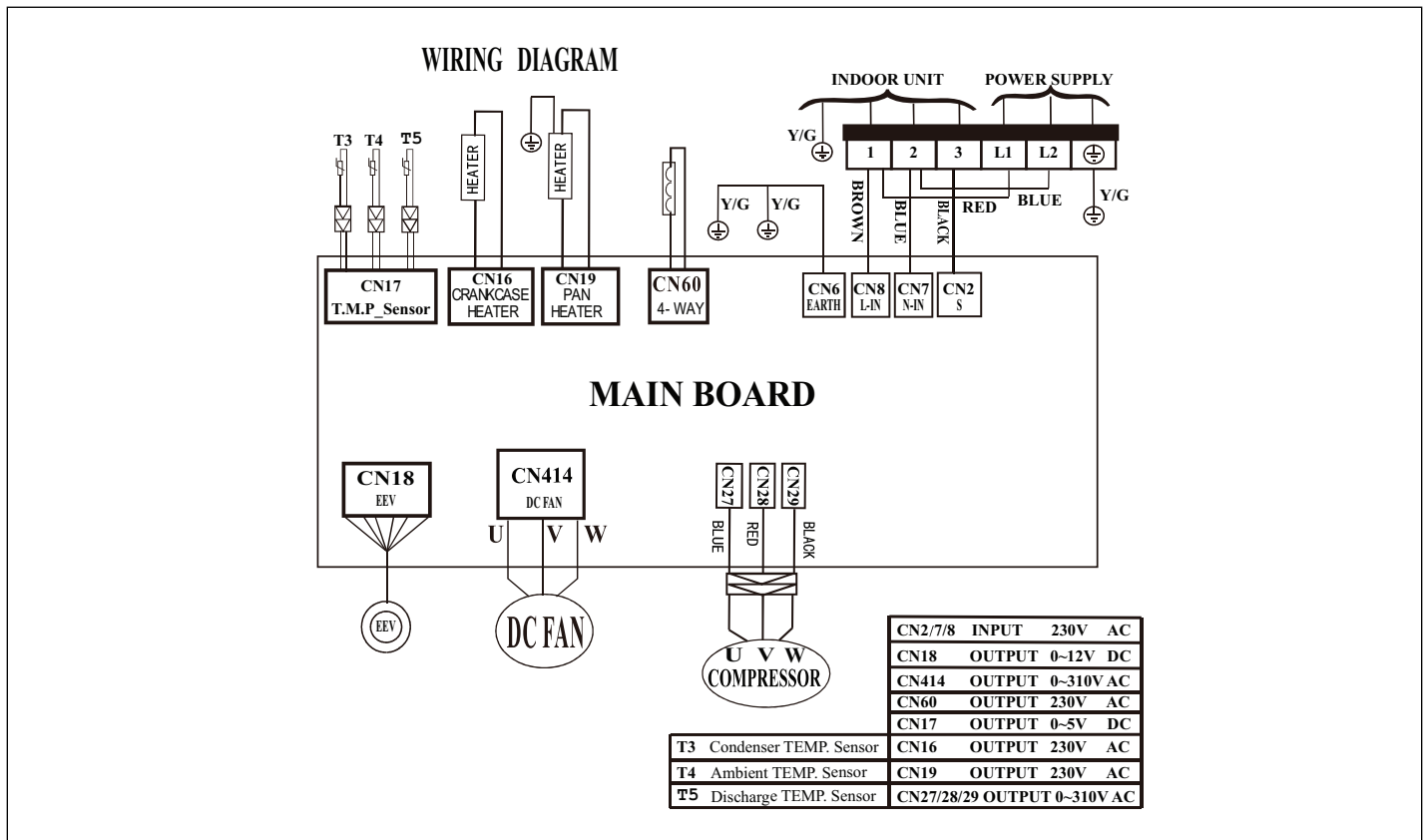
Figure 44. Schéma de câblage de l'unité extérieure 208/230V MPC018S4S-*P
