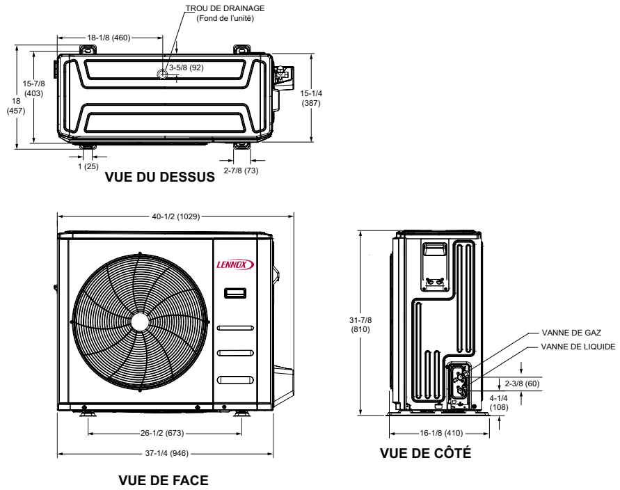
Figure 8. MLB024S4S-*P - Dimensions de l'unité - pouces (mm)
