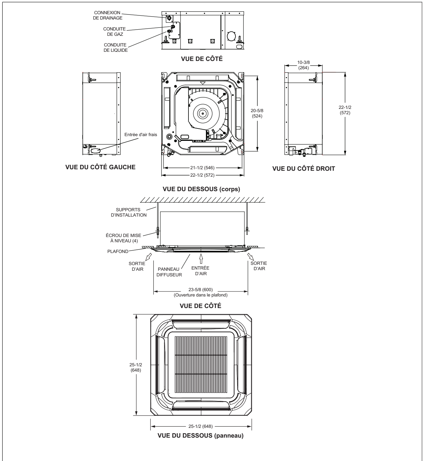
Figure 10. Dimensions des unités intérieures à cassette M22A - pouces (mm)
