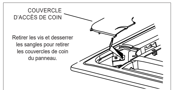
Figure 17. Retirer les couvercles de coin
