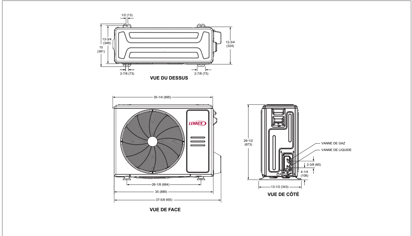
Figure 3. MPC018S4S-*P - Dimensions de l'unité - pouces (mm)
