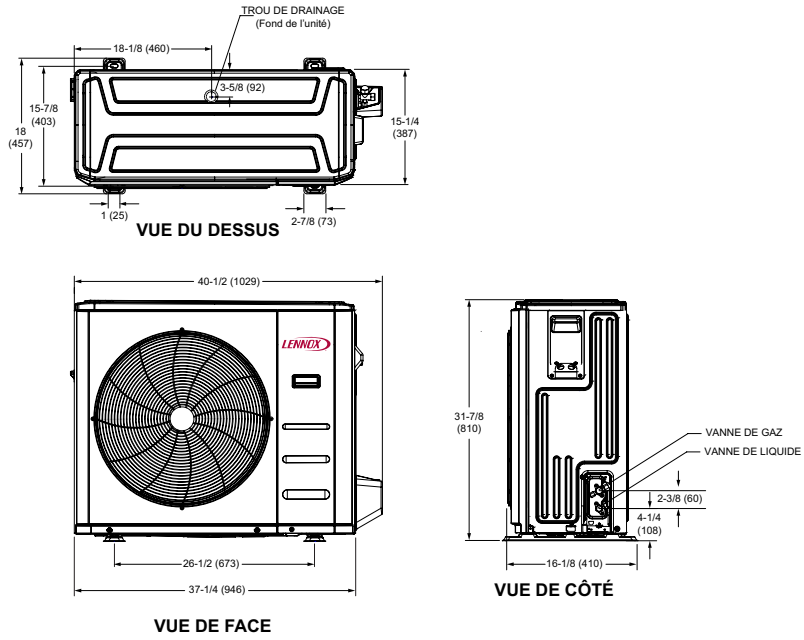
Figure 4. MPC024S4S-*P et MPC036S4S-*P - Dimensions de l'unité - pouces (mm)
