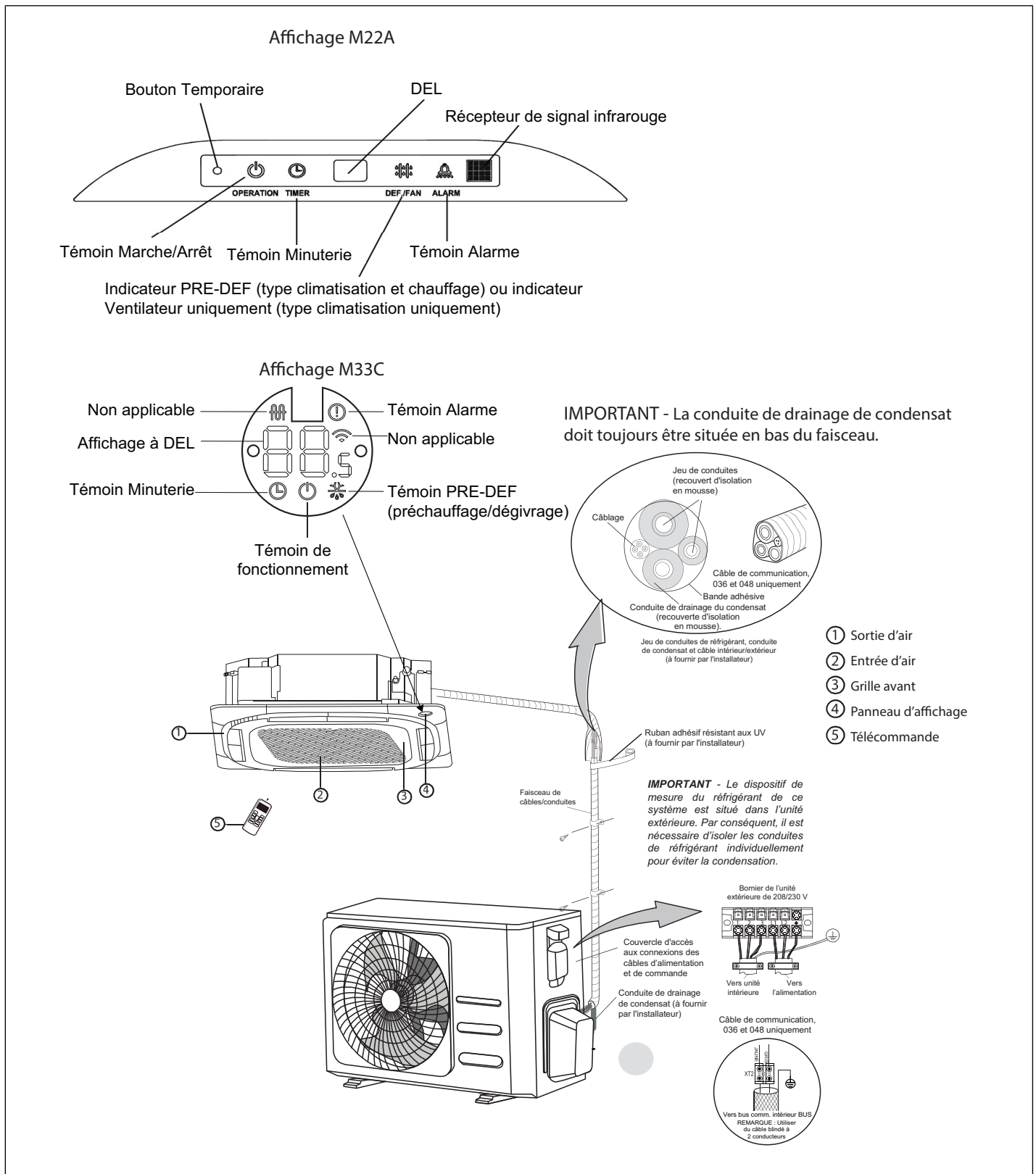
Figure 1. Système M33C simple zone typique illustré
