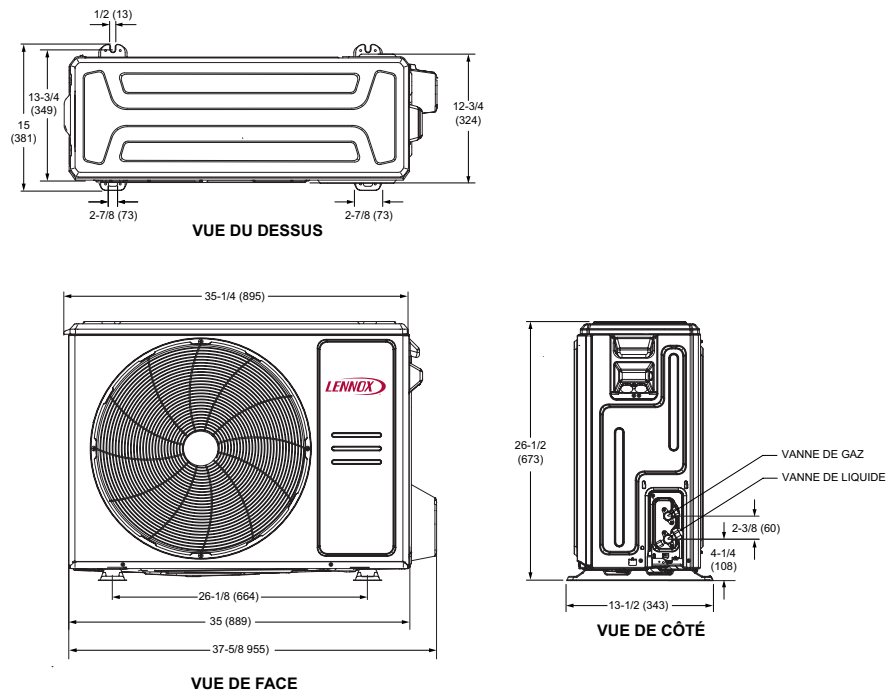
Figure 7. MLB018S4S-*P - Dimensions de l'unité - pouces (mm)
