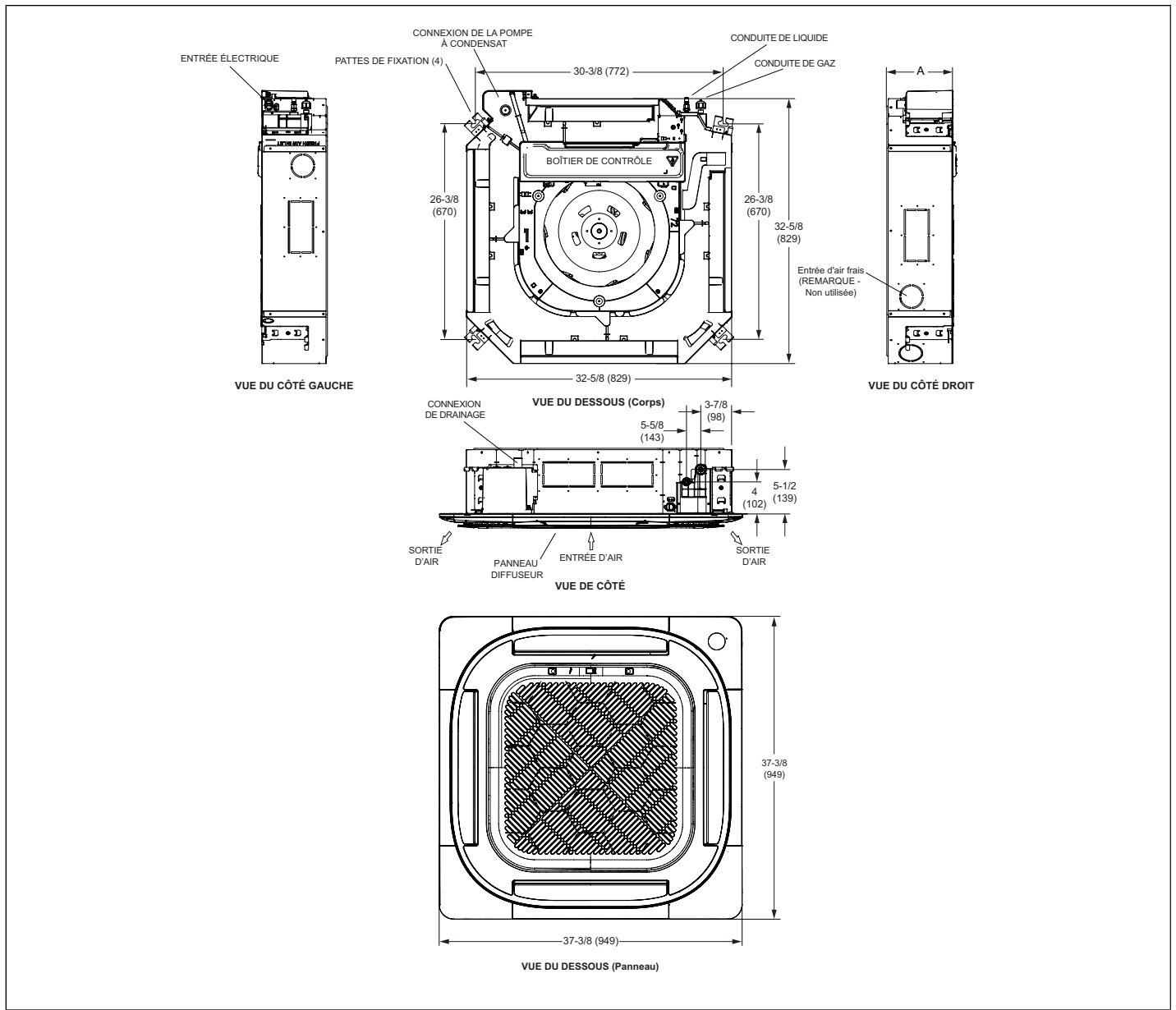
Figure 11. Dimensions des unités intérieures à cassette M33C - pouces (mm)
