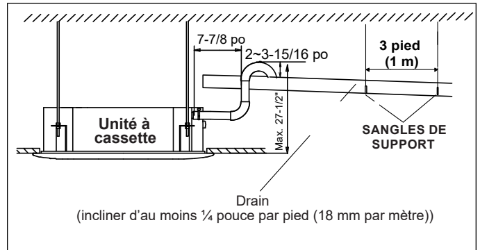
Figure 22. Drainage du condensat de l'unité intérieure
