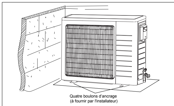
Figure 32. Fixation de l'unité extérieure sur une dalle
