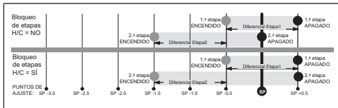
Imagen 3. Calefacción: sin bomba de calor o bomba de calor con calefacción de respaldo: etapas 1 o 2
