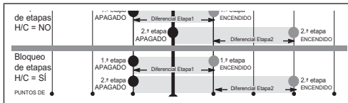
Imagen 2. Etapas 1 o 2 de enfriamiento
