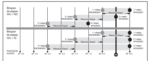
Imagen 4. Calefacción: bomba de calor eléctrica: etapa 3 (2 compresores/1 respaldo) O 1 compresor/2 respaldos)
