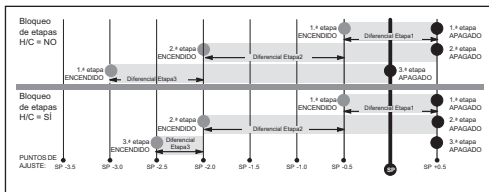
Imagen 7. Calefacción: bicombustible: etapa 3 (1 compresor/2 respaldos)
