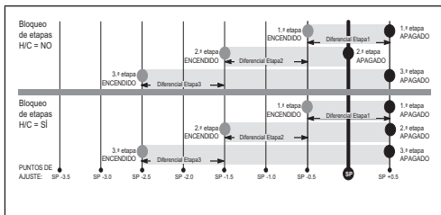
Imagen 8. Calefacción: bicombustible: etapa 3 (2 compresores/1 respaldo)
