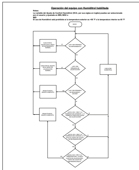
Imagen 10. Operación del equipo con Humiditrol habilitada
