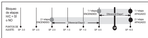
Imagen 6. Calefacción: bicombustible: etapa 2 (1 compresor/1 respaldo)
