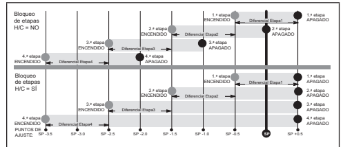
Imagen 5. Calefacción: bomba de calor eléctrica: etapa 4 (2 compresores/2 respaldos)
