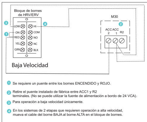
Imagen 11. Cableado de ERV / HRV
