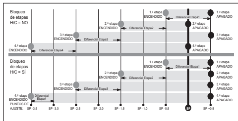
Imagen 9. Calefacción: bicombustible: etapa 4 (2 compresores/2 respaldos)
