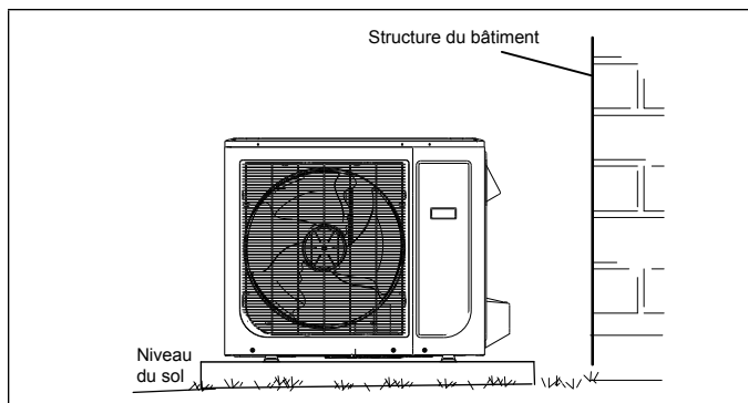
Figure 12. Installer l'unité de niveau (horizontale)
