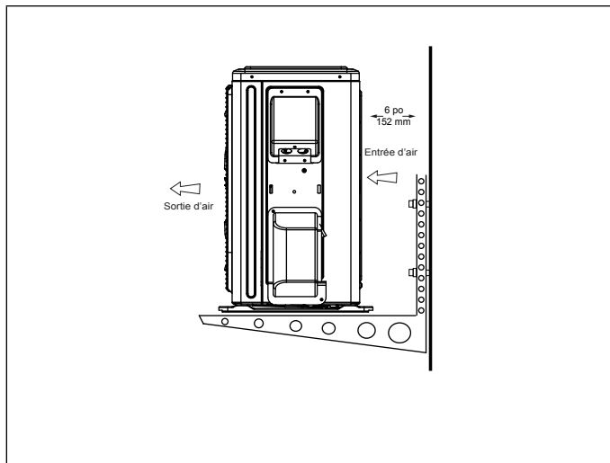
Figure 23. Fixation de l'unité extérieure sur des équerres
