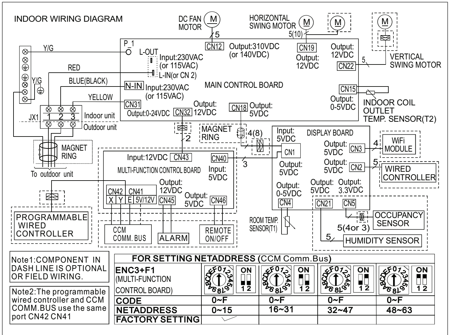
Figure 28. Schéma de câblage de l'unité intérieure 3WMC036
