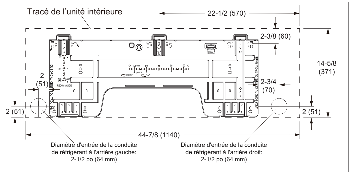
Figure 4. Dimensions de la plaque murale de l'unité intérieure - pouces (mm)
