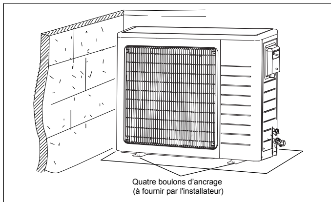
Figure 21. Fixation de l'unité extérieure sur une dalle
