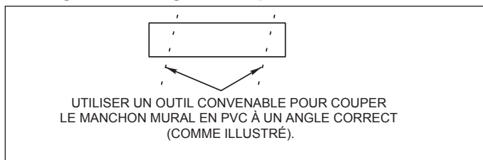
Figure 9. Installation du manchon mural en PVC
