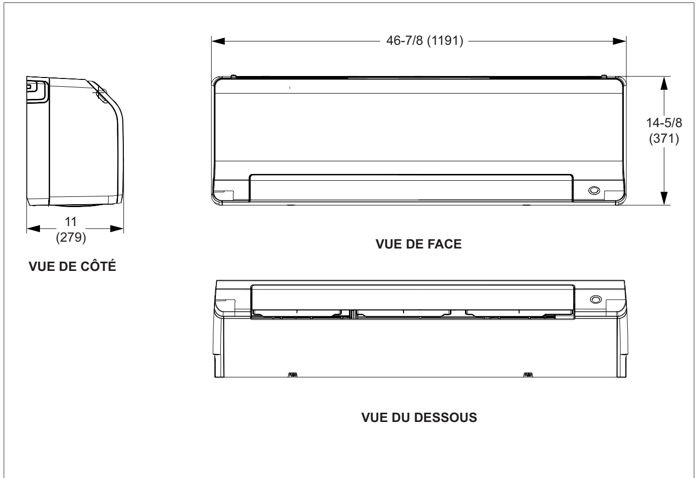
Figure 3. Dimensions de l'unité intérieure - pouces (mm)
