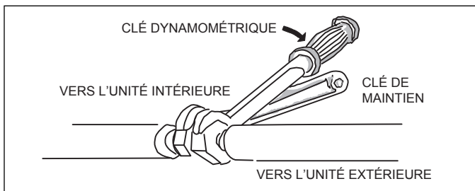
Figure 26. Serrer l'écrou évasé
