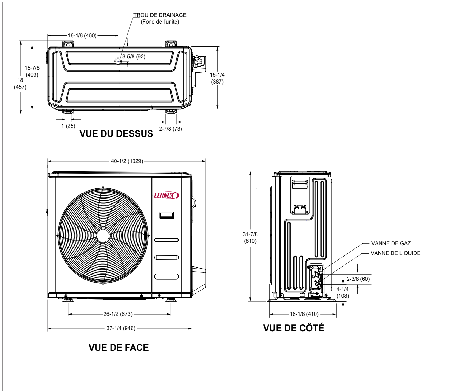
Figure 2. 3PC036S4S-1P - Dimensions de l'unité extérieure - pouces (mm)
