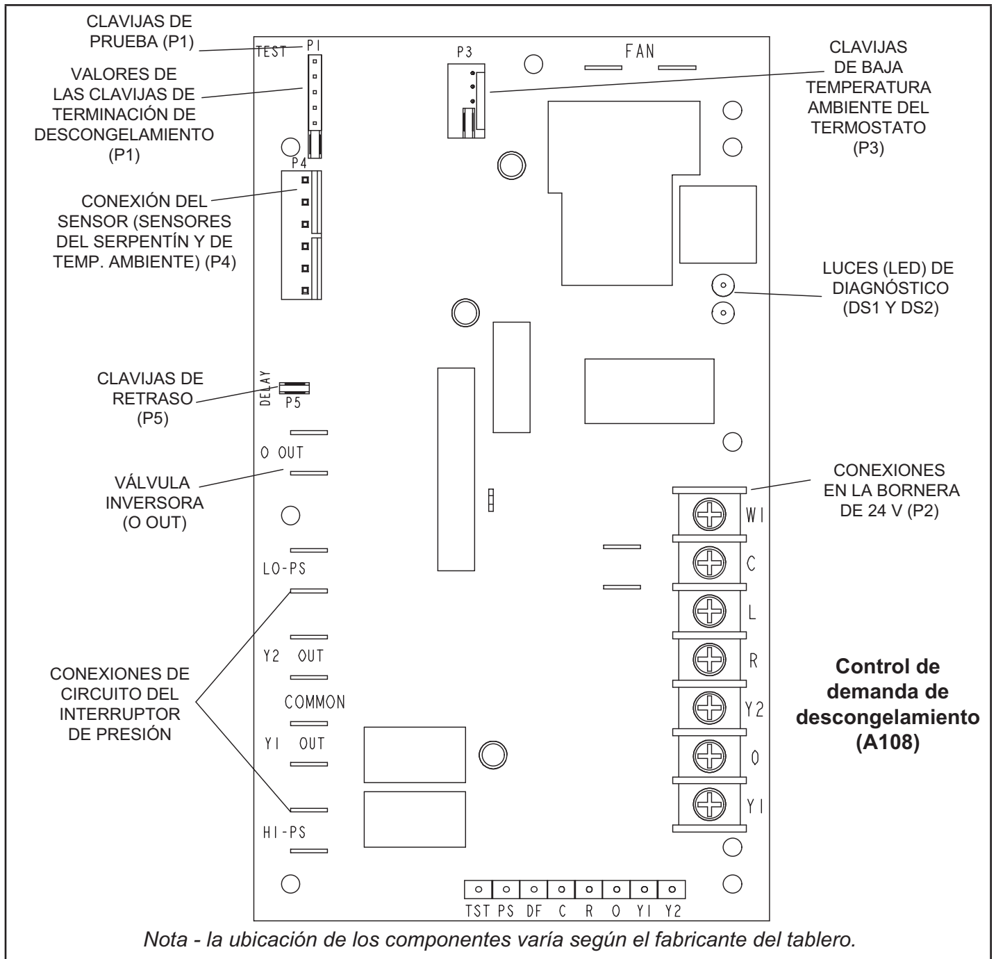
FIGURA 18. Control de demanda de descongelamiento
