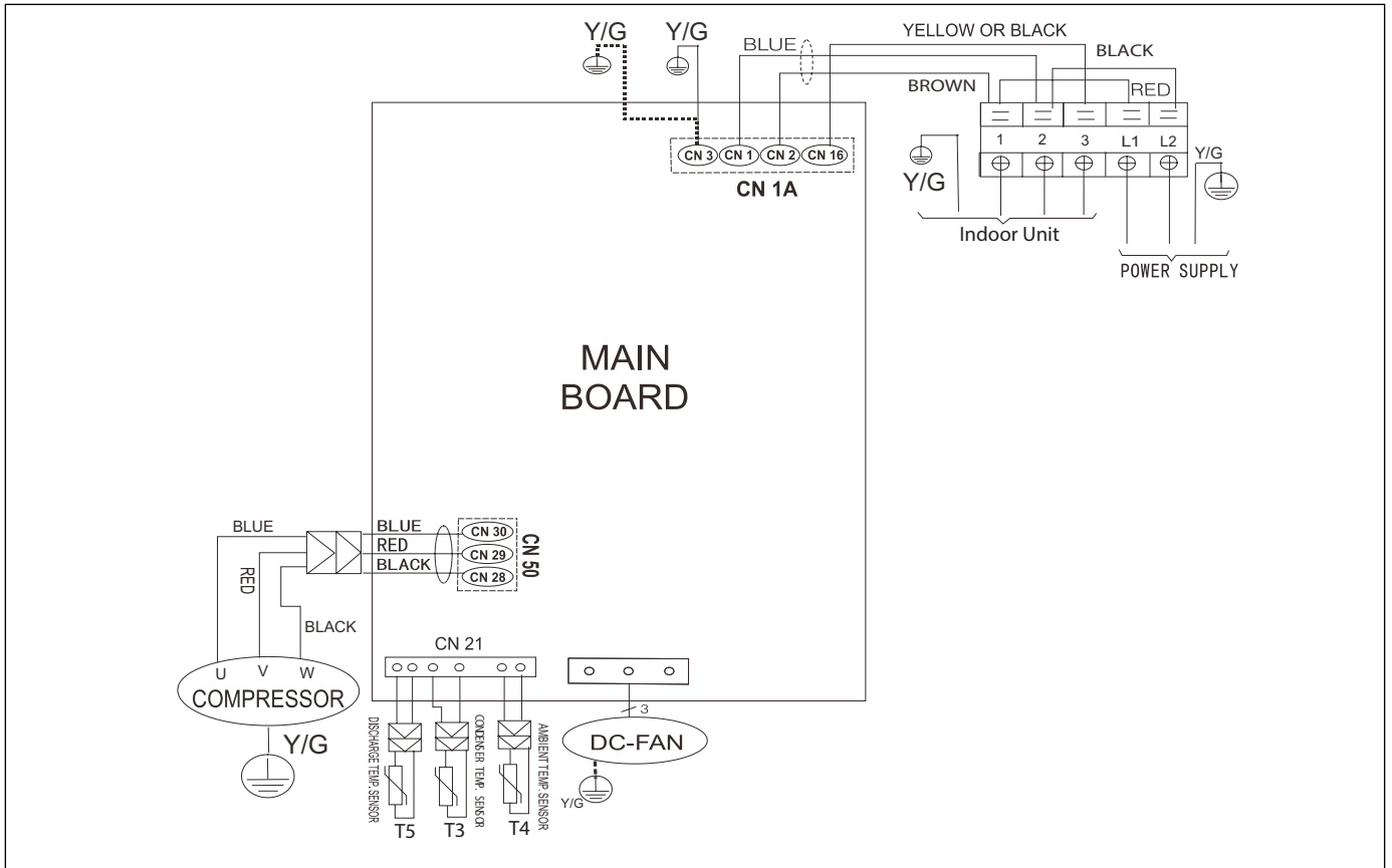
Figure 29. 09 et 12K - Schéma de câblage de l'unité extérieure 208/230 VCA
