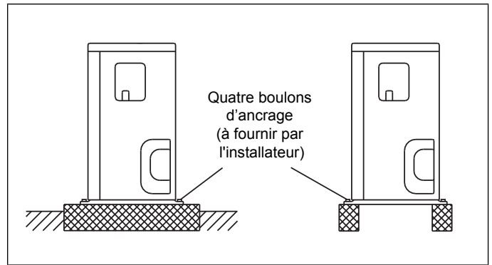
Figure 21. Fixation de l'unité extérieure sur des rails
