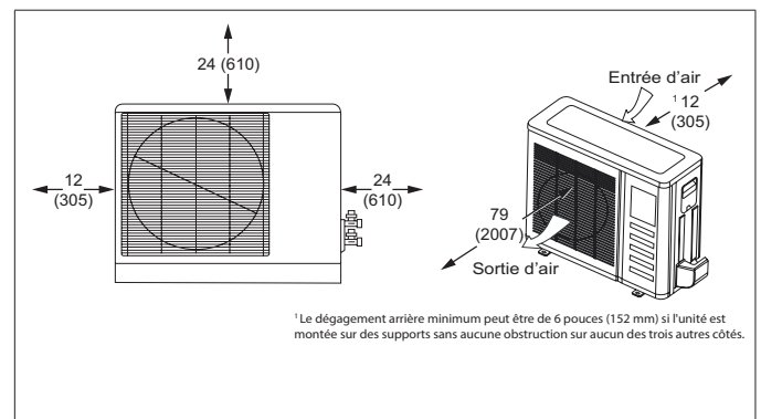
Figure 9. Dégagements de l'unité extérieure - pouces (mm)
