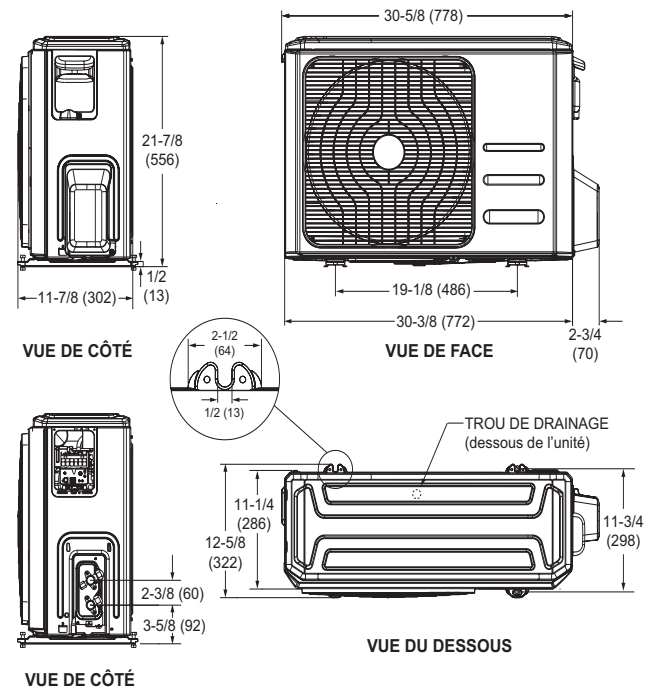
Figure 2. 09, 12K et 18K - Dimensions des unités extérieures - pouces (mm)
