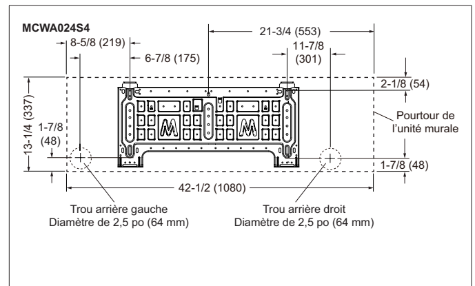
Figure 8. 24K - Dimensions de la plaque murale de l'unité intérieure - pouces (mm)
