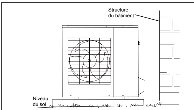
Figure 17. Installer l'unité de niveau (horizontale)
