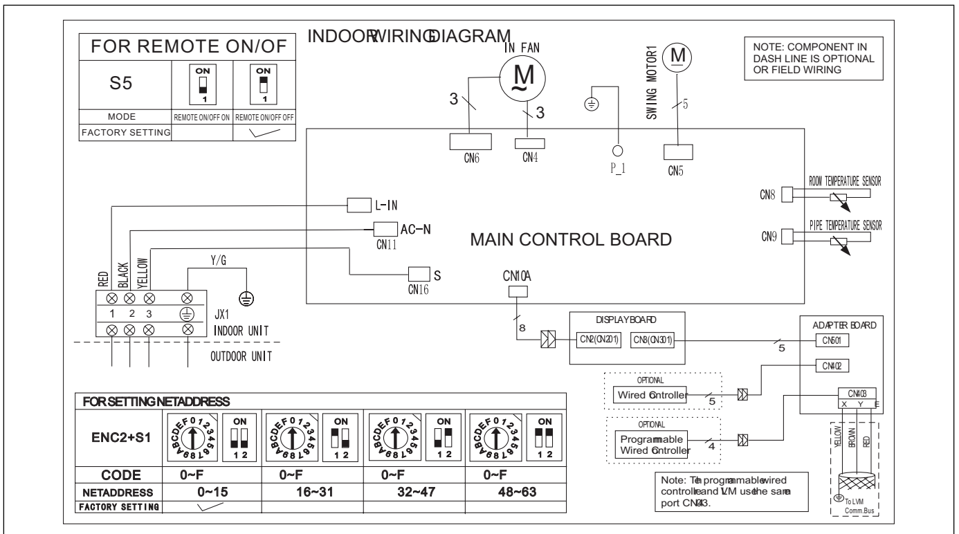
Figure 32. 09K et 12K - Schéma de câblage de l'unité intérieure (115 et 208/230 VCA)
