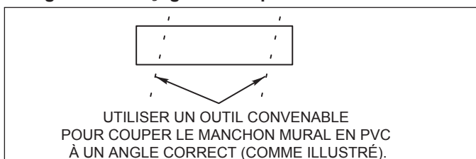
Figure 14. Installation du manchon mural en PVC
