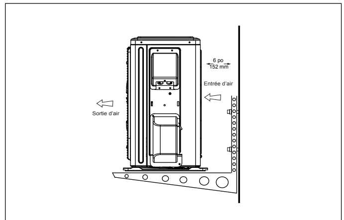
Figure 22. Fixation de l'unité extérieure sur des équerres
