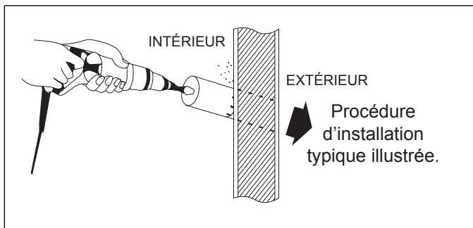
Figure 13. Perçage du trou pour le manchon mural
