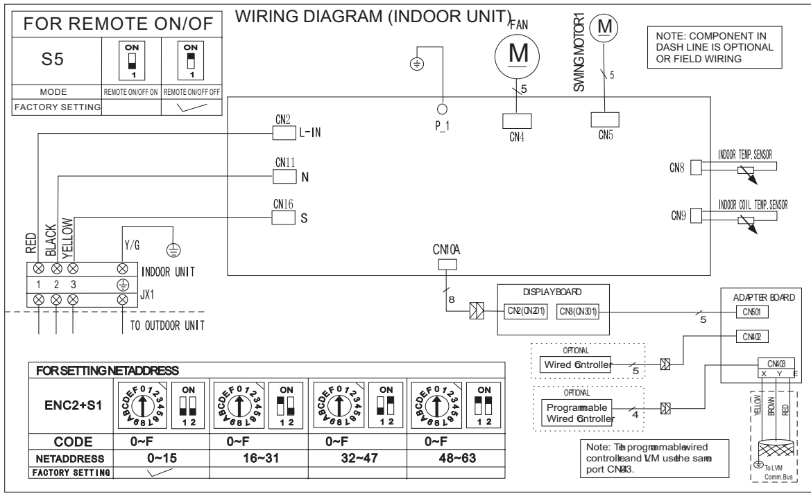
Figure 33. 18K - Schéma de câblage de l'unité intérieure 208/230 VCA
