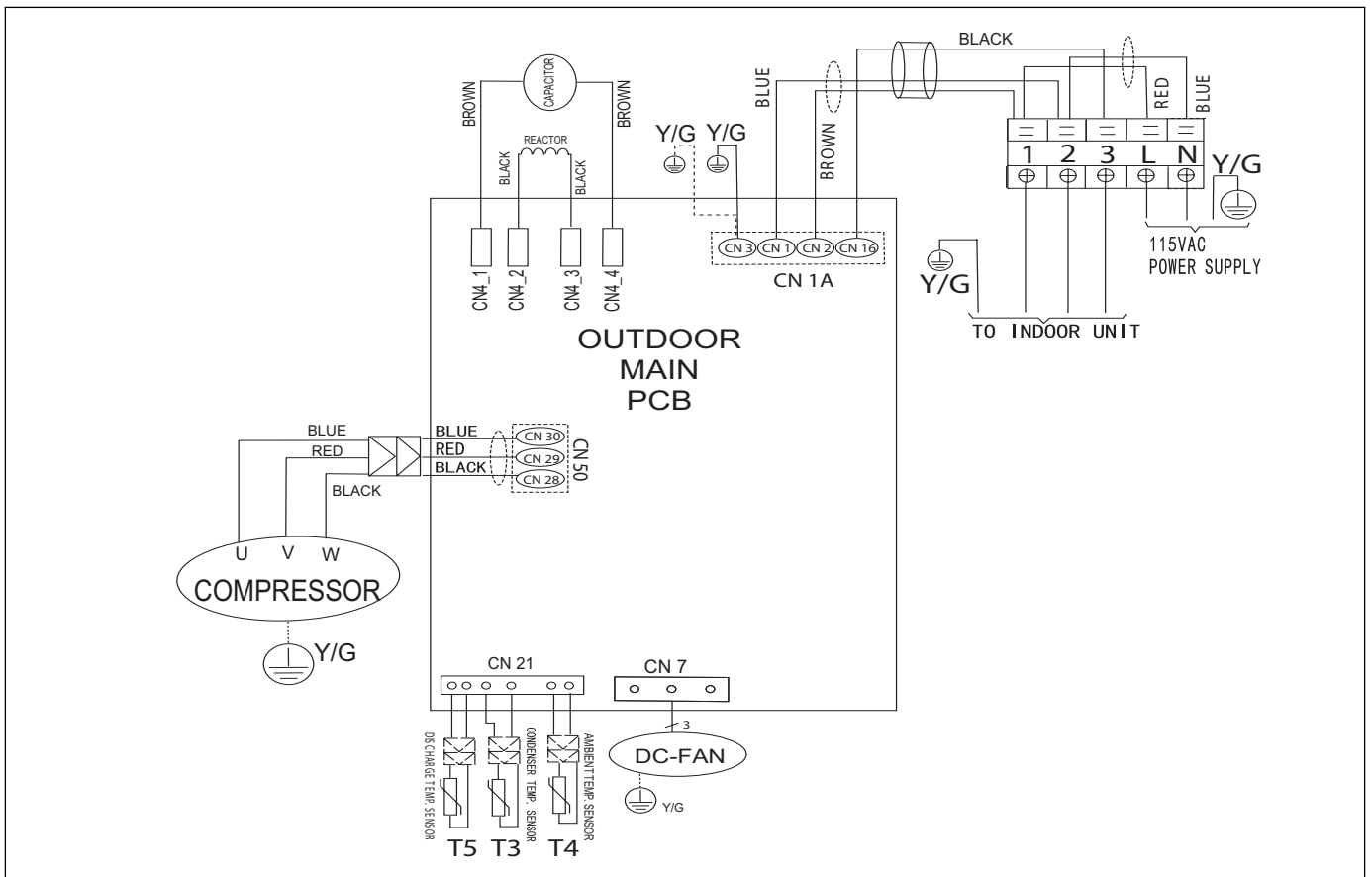
Figure 30. 12K - Schéma de câblage de l'unité extérieure 115 VCA
