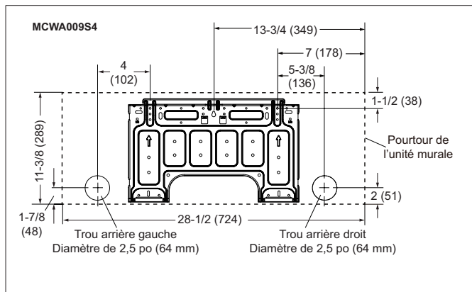
Figure 5. 9K - Dimensions de la plaque murale de l'unité intérieure - pouces (mm)
