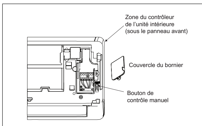
Figure 35. Bouton de contrôle manuel
