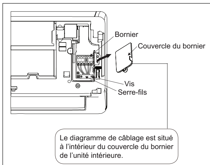
Figure 27. Bornier de l'unité intérieure
