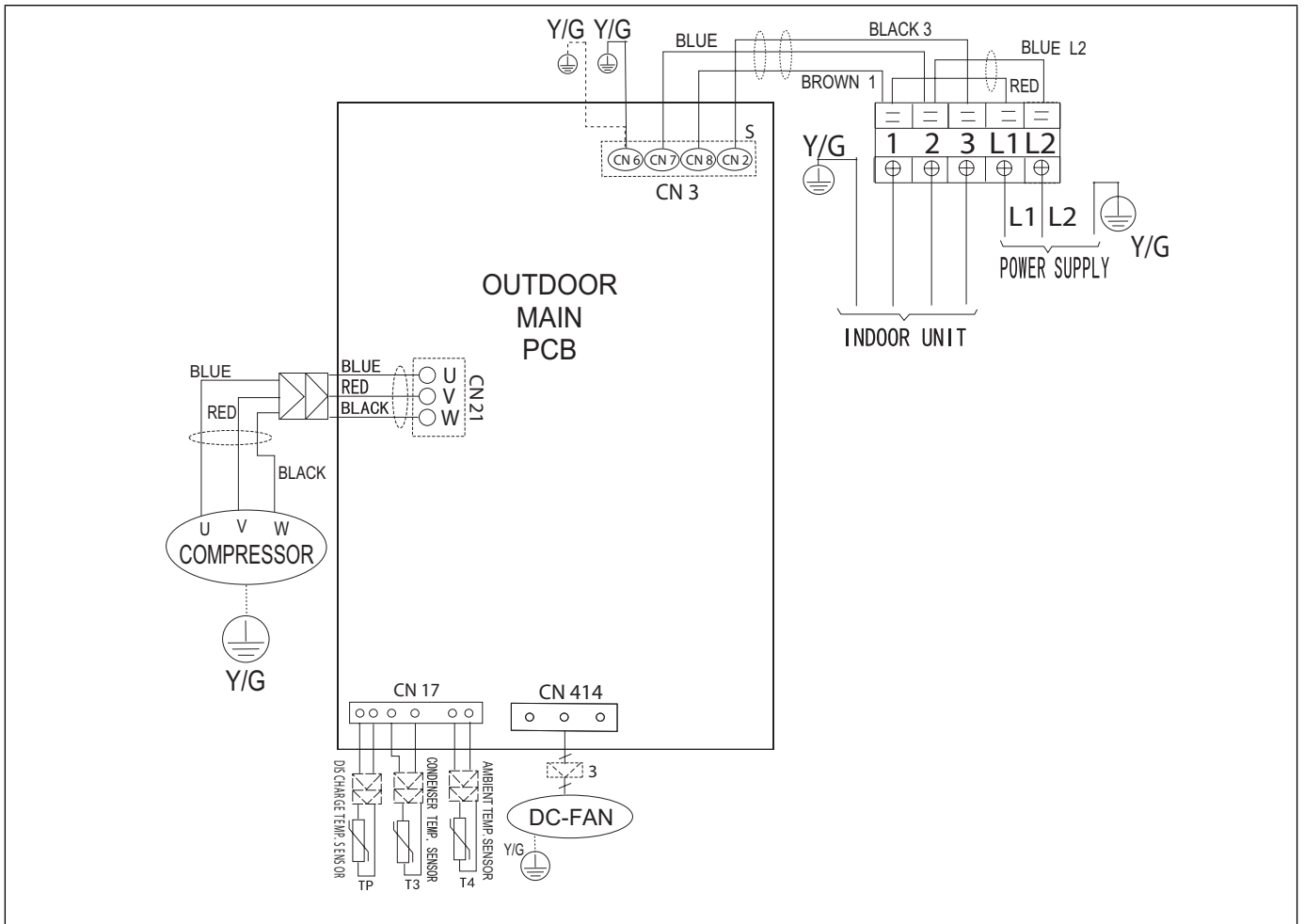
Figure 31. 18K et 24K - Schéma de câblage de l'unité extérieure 208/230 VCA
