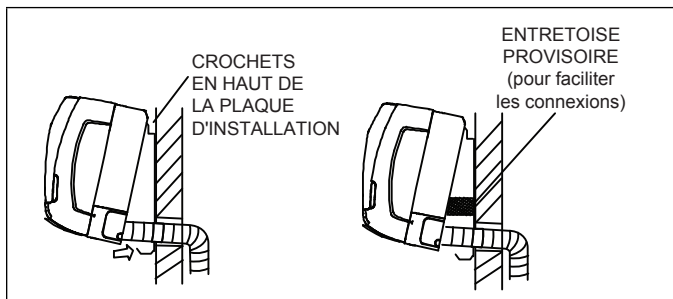
Figure 15. Fixation de l'unité sur la plaque d'installation murale
