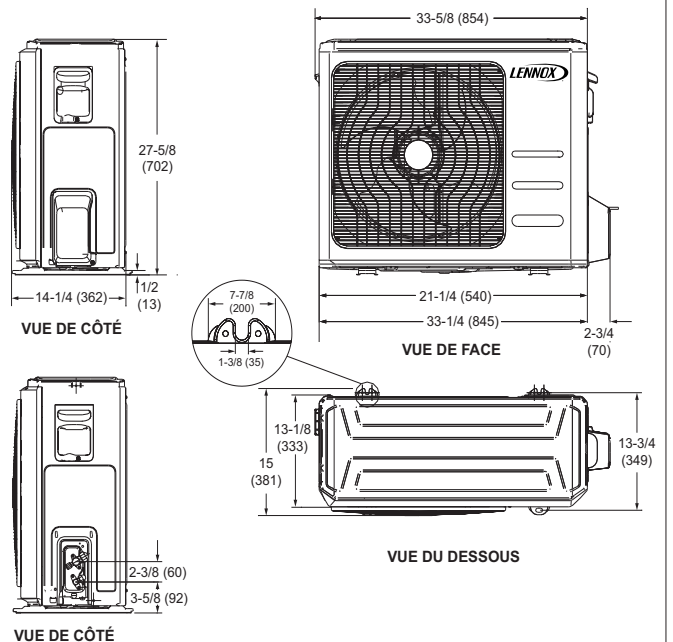
Figure 3. 24K - Dimensions de l'unité extérieure - pouces (mm)
