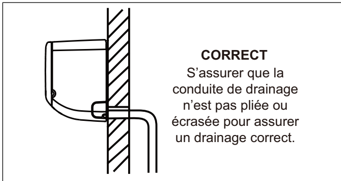
Figure 16. Conduite de condensat
