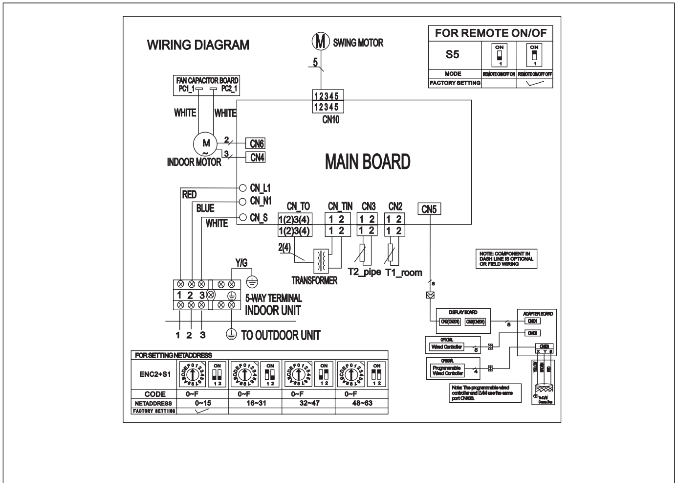
Figure 34. 24K - Schéma de câblage de l'unité intérieure 208/230 VCA
