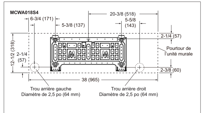
Figure 7. 18K - Dimensions de la plaque murale de l'unité intérieure - pouces (mm)
