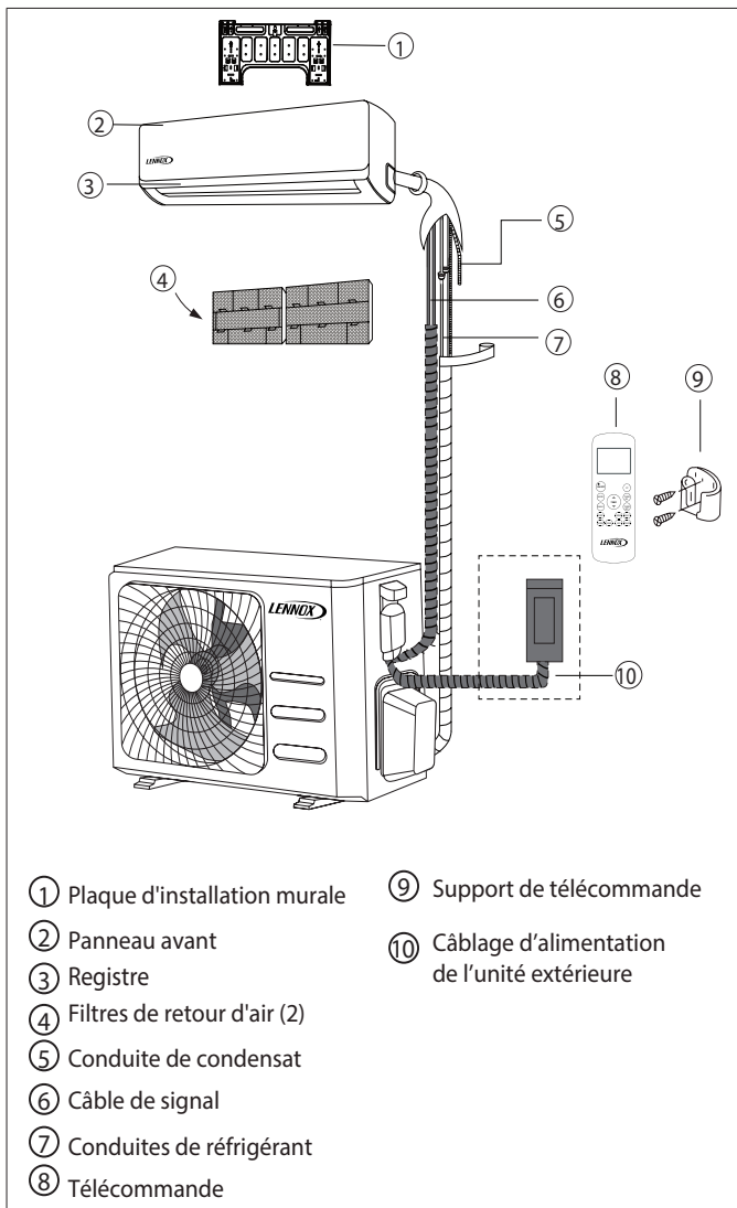
Figure 1. Système typique illustré
