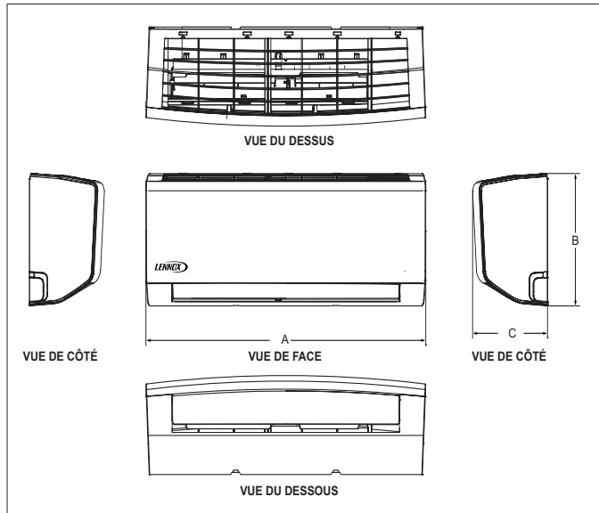
Figure 4. Dimensions de l'unité intérieure - pouces (mm)
