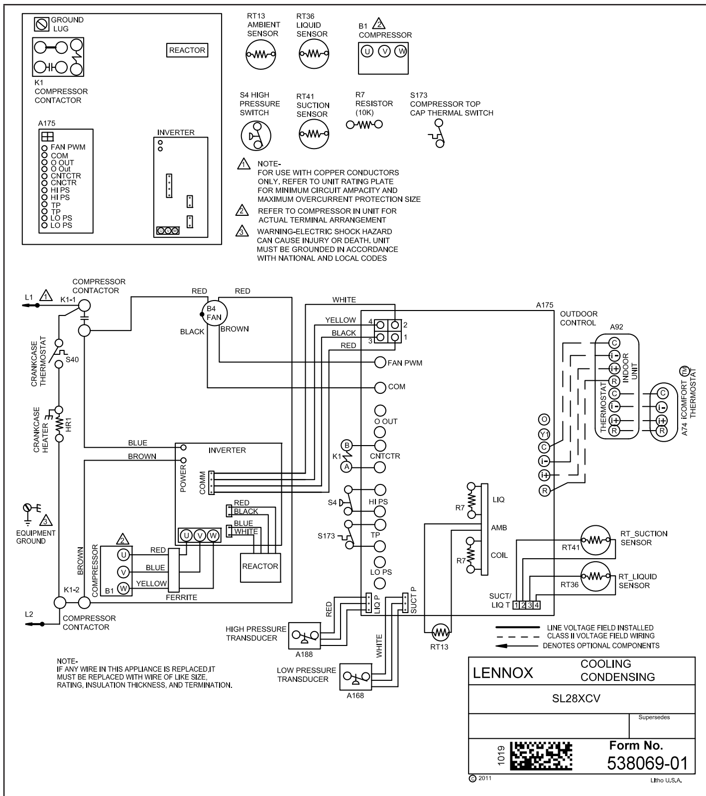
FIGURA 10. Cableado típico en el sitio
