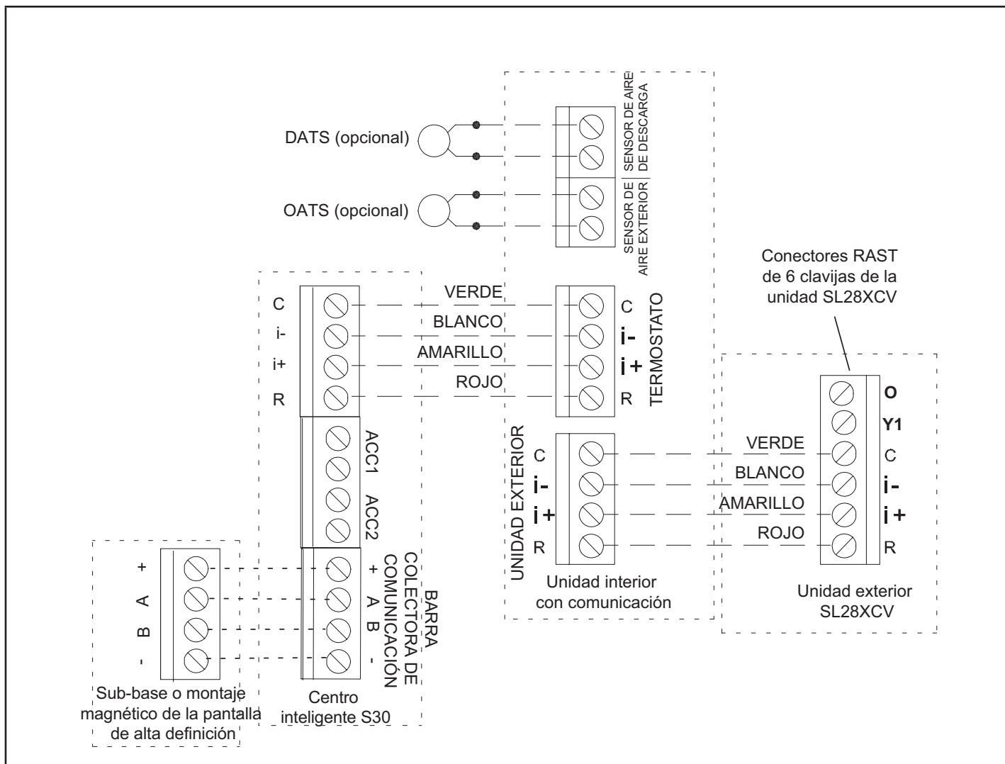
FIGURA 12. SL28XCV con termostato iComfort S30 con comunicación – Diagrama de cableado en el sitio
