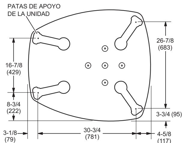
BASE CON SOPORTES ALARGADOS
