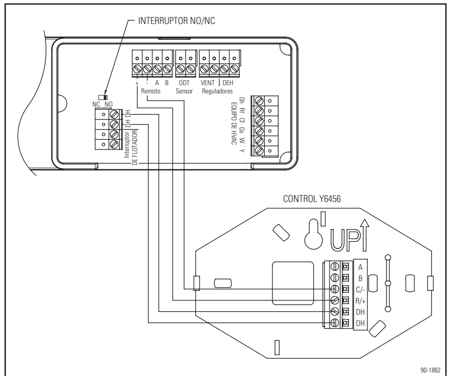
Figura 23. Cableado de control externo Y6456
