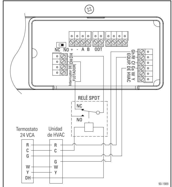
Figura 21. Conexiones de termostato de 24 VCA
