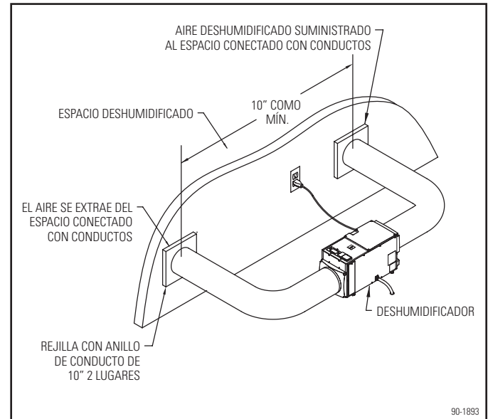
Figura 16. Instalación independiente con conexión de conductos
