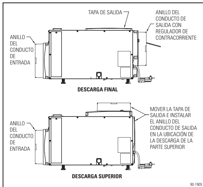
Figura 2. Instalaciones con conexión completa de conductos
