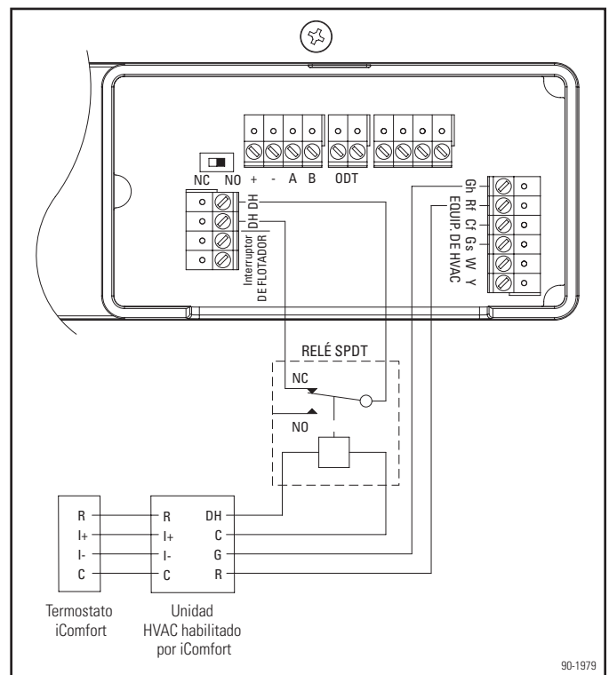
Figura 22. Conexiones de termostato de comunicación
