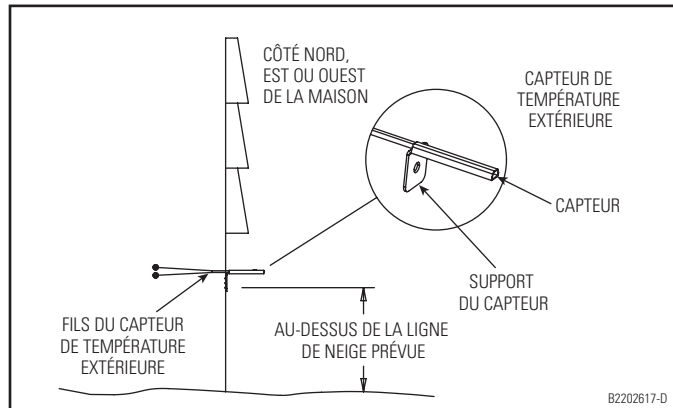
Figure 30. Capteur de température extérieure installé à l'extérieur
