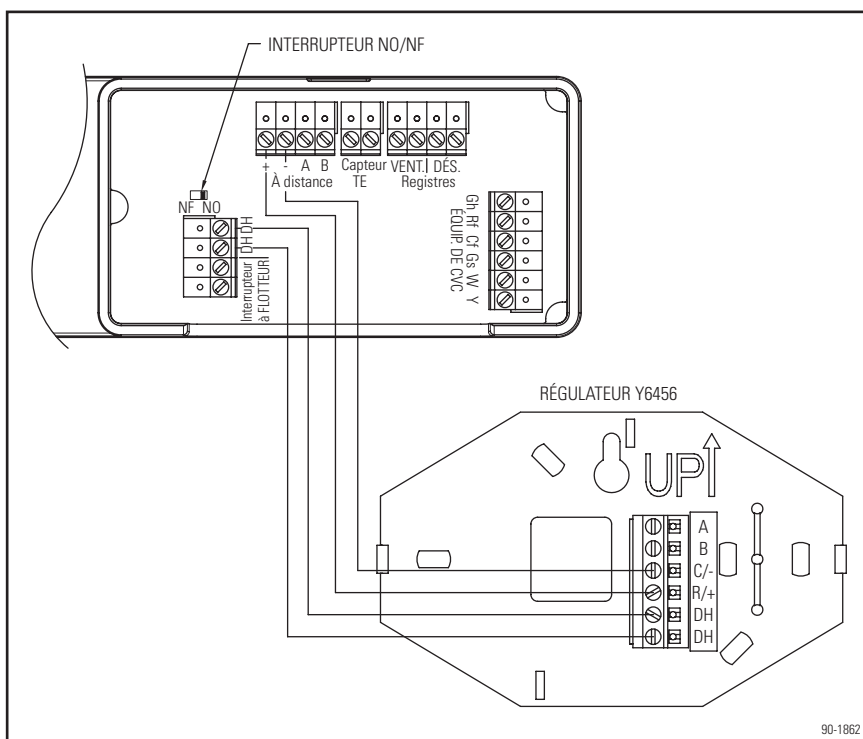
Figure 23. Câblage du régulateur externe Y6456
