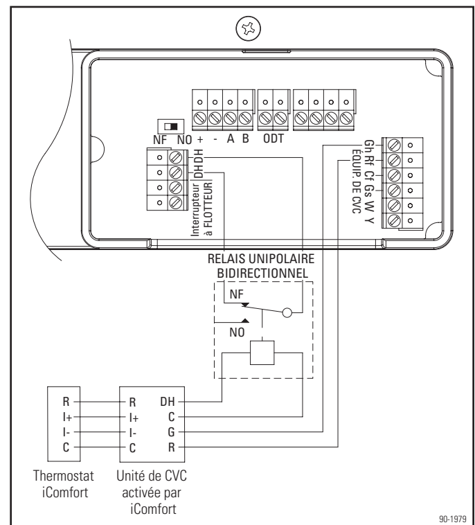
Figure 22. Connexions du thermostat de communication
