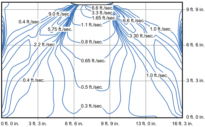
V33B036 - COOLING
